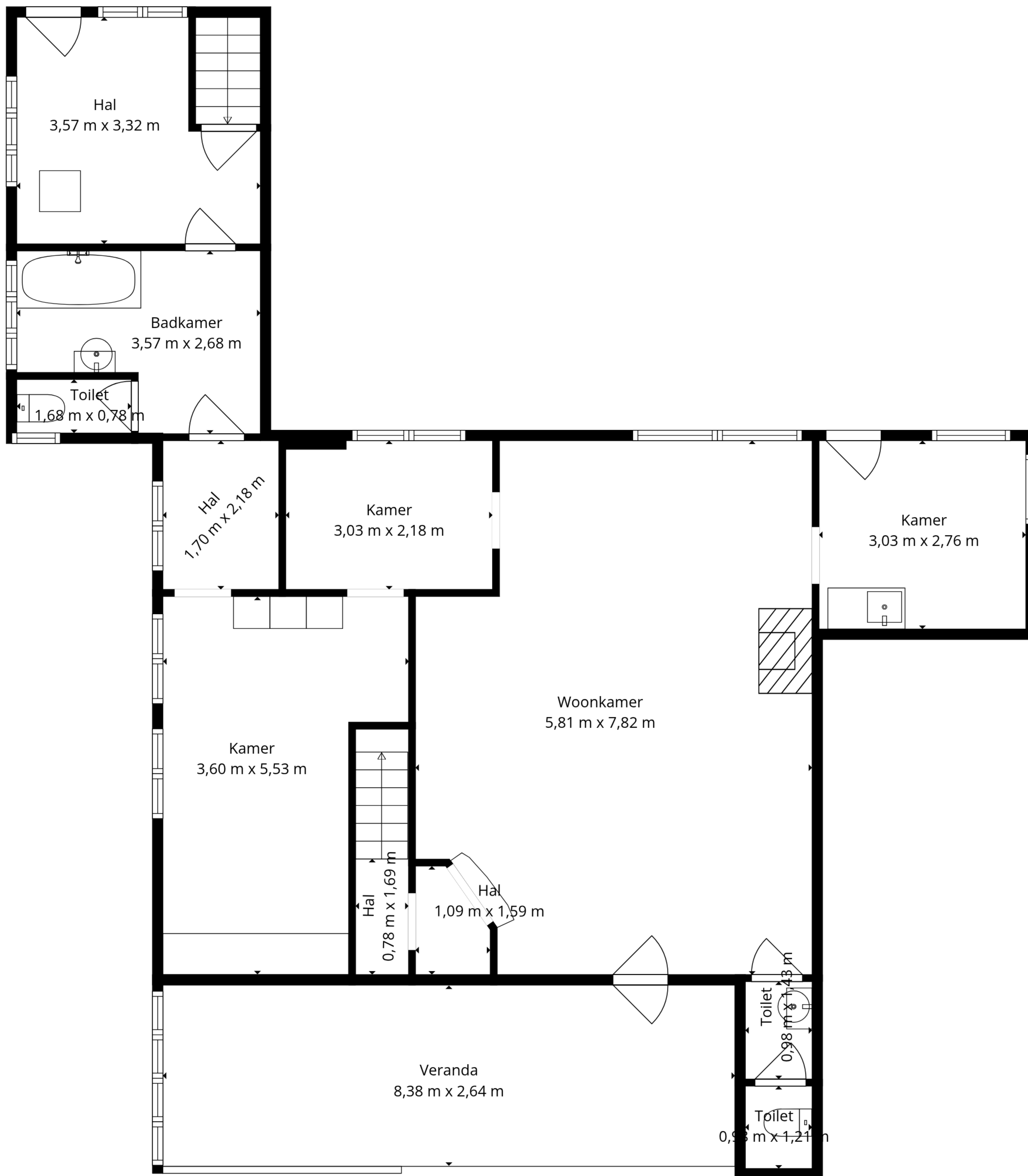
1e Verdieping
