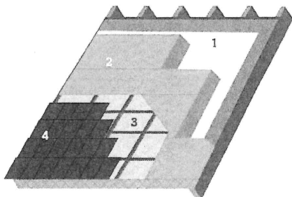
1. Damperscreen | 2. Isolatie | 3. Onderdak | 4. Dakbedekking
