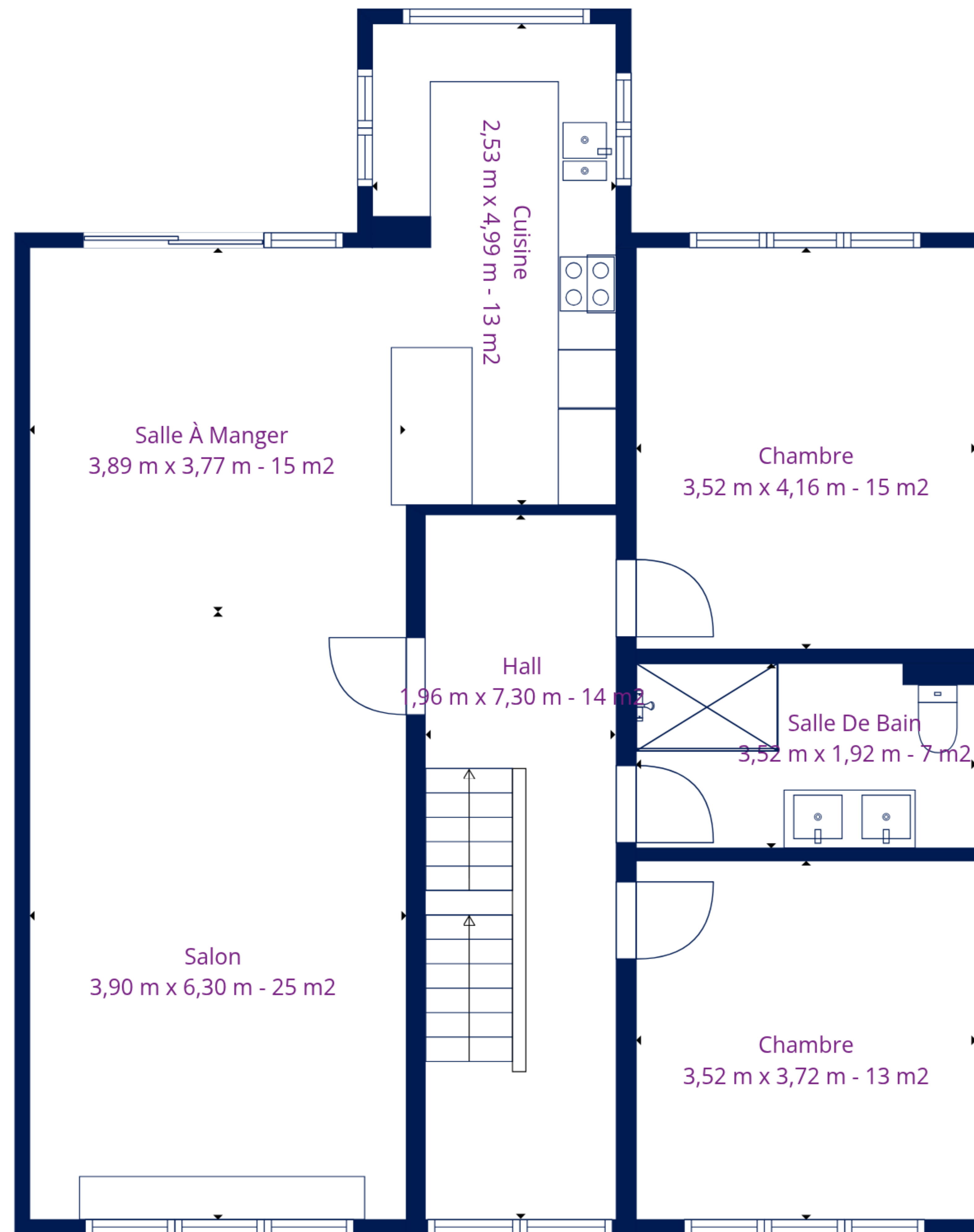
Rez-de-chaussée
