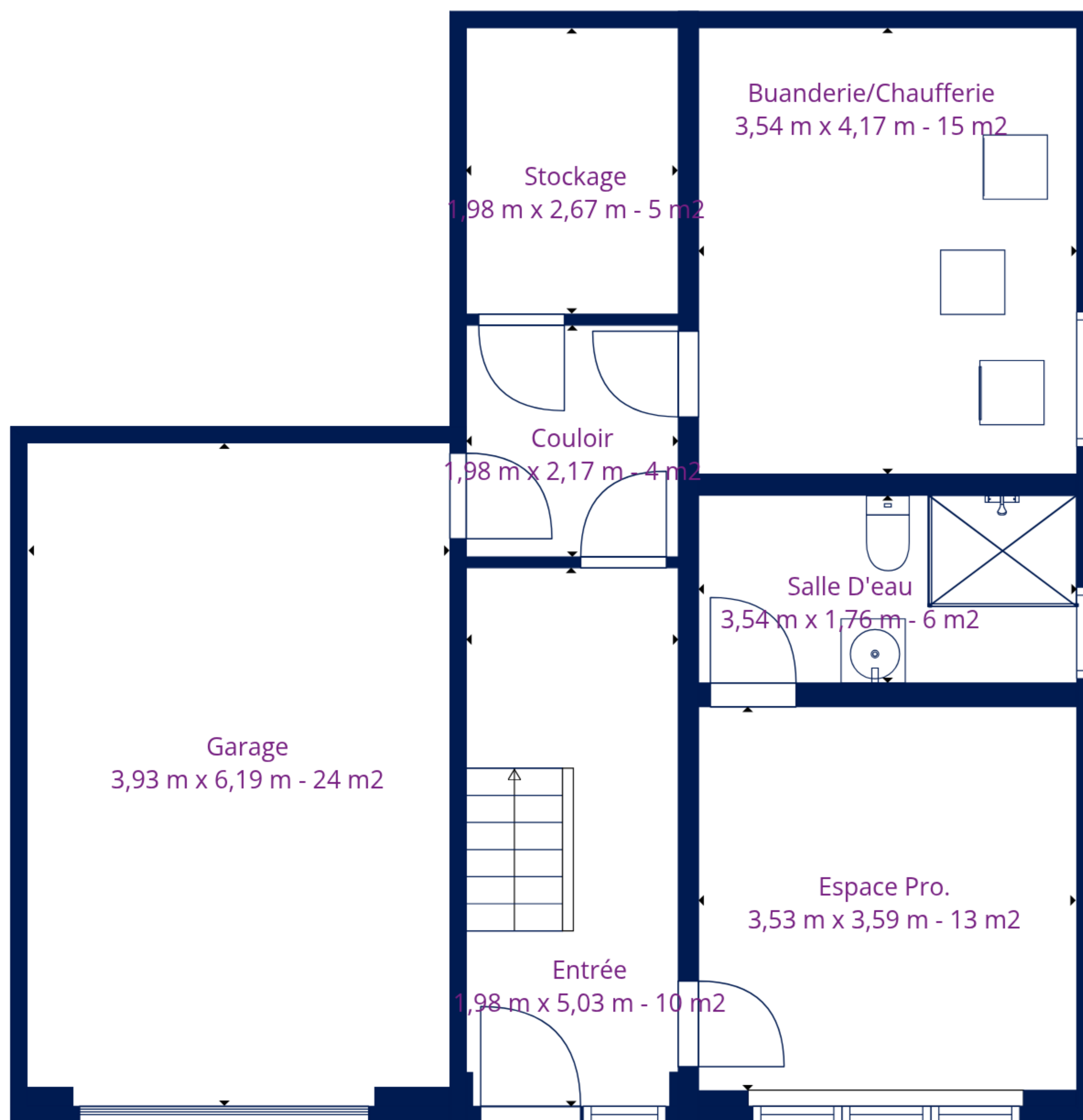
Sous-sol
