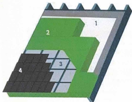
1. Dampscherm | 2. Isolatie | 3. Onderdak | 4. Dakbedekking
