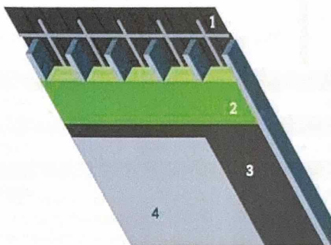
1. Onderdak | 2. Isolatie | 3. Dampscherm | 4. binnenafwerking
