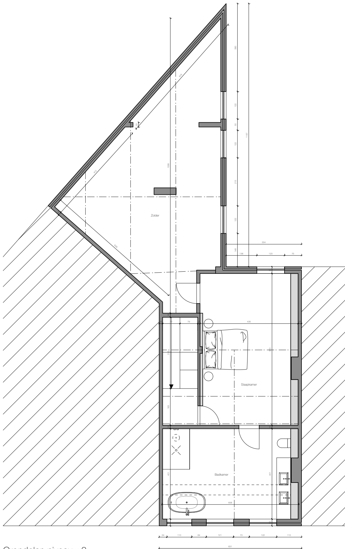
Grondplan niveau +2 Leopoldstraat 9a, 2300 Turnhout schaal 1:100
