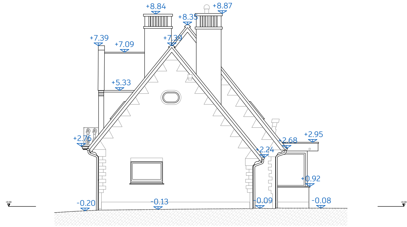
GEVEL RECHTS
