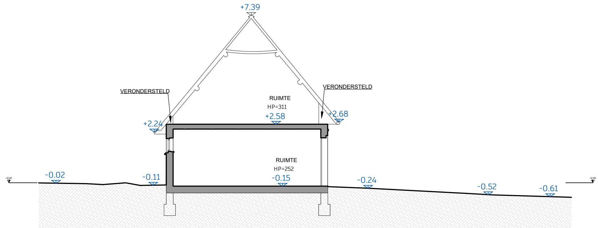
SNEDE C
