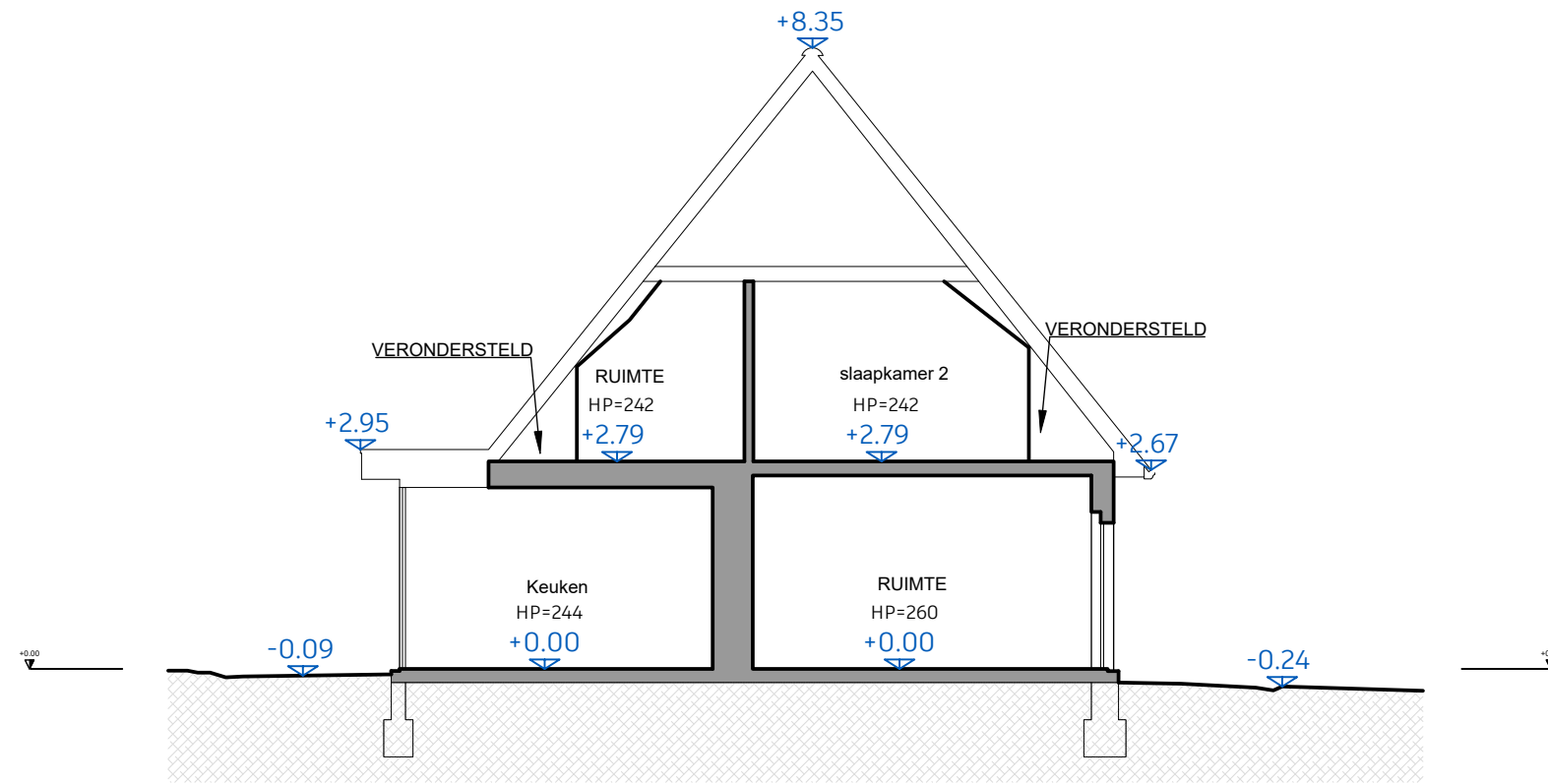
SNEDE B
