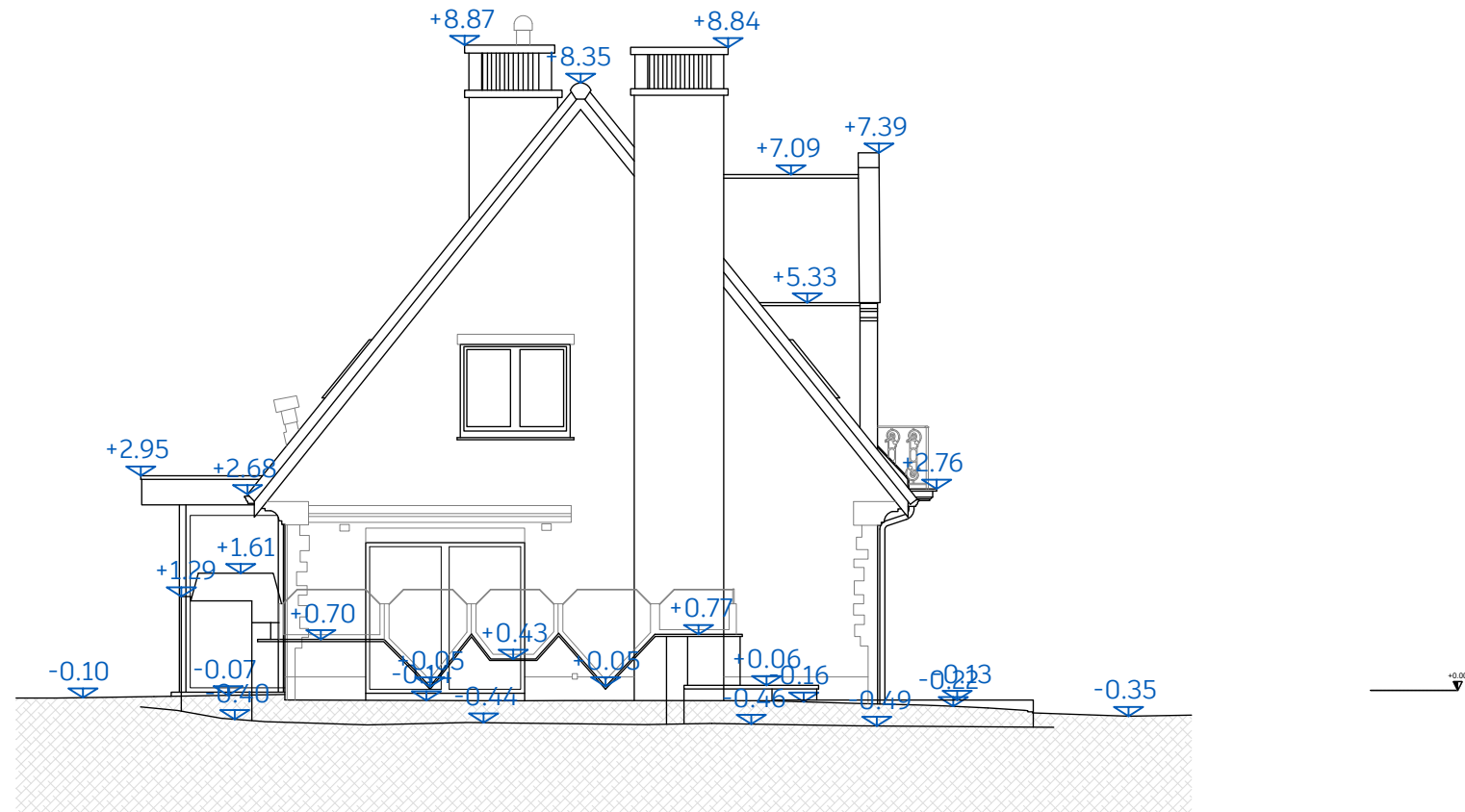
GEVEL LINKS
