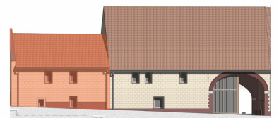
GEVEL Visesteenweg
