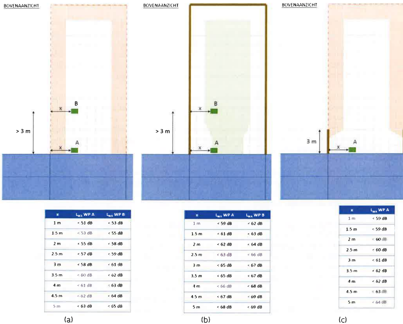
Figuur 15: Maximale geluidsvermogniveaus van de buitenunit voor diverse posities in de achtertuin (positie A en B 35 ) om te voldoen aan de vooropgestelde geluidsvoorwaarde 45 dB(A) L Aeq,1min overdag. x is de kleinste afstand tot de dichtstbijzijnde perceelsgrens. De geluidsbron wordt verondersteld op 0,75 m (2/3 van de hoogte van de unit) en de geluidsdruk werd geëvalueerd op de perceelsgrens op 1,5 m hoogte. In situatie (a) zijn geen afsluitingen tussen de tuinen die een voldoende massa hebben om te zorgen voor afscherming. In situatie (b) is een volledig gesloten afsluiting met hoogte 1,8m en oppervlaktemassa \geq 10\text{kg/m}^2 rondom de volledige tuin 36 en in situatie (c) zijn volledig gesloten afsluitingen met lengte 3 m, hoogte 1,8 m en oppervlaktemassa \geq 10\text{kg/m}^2
