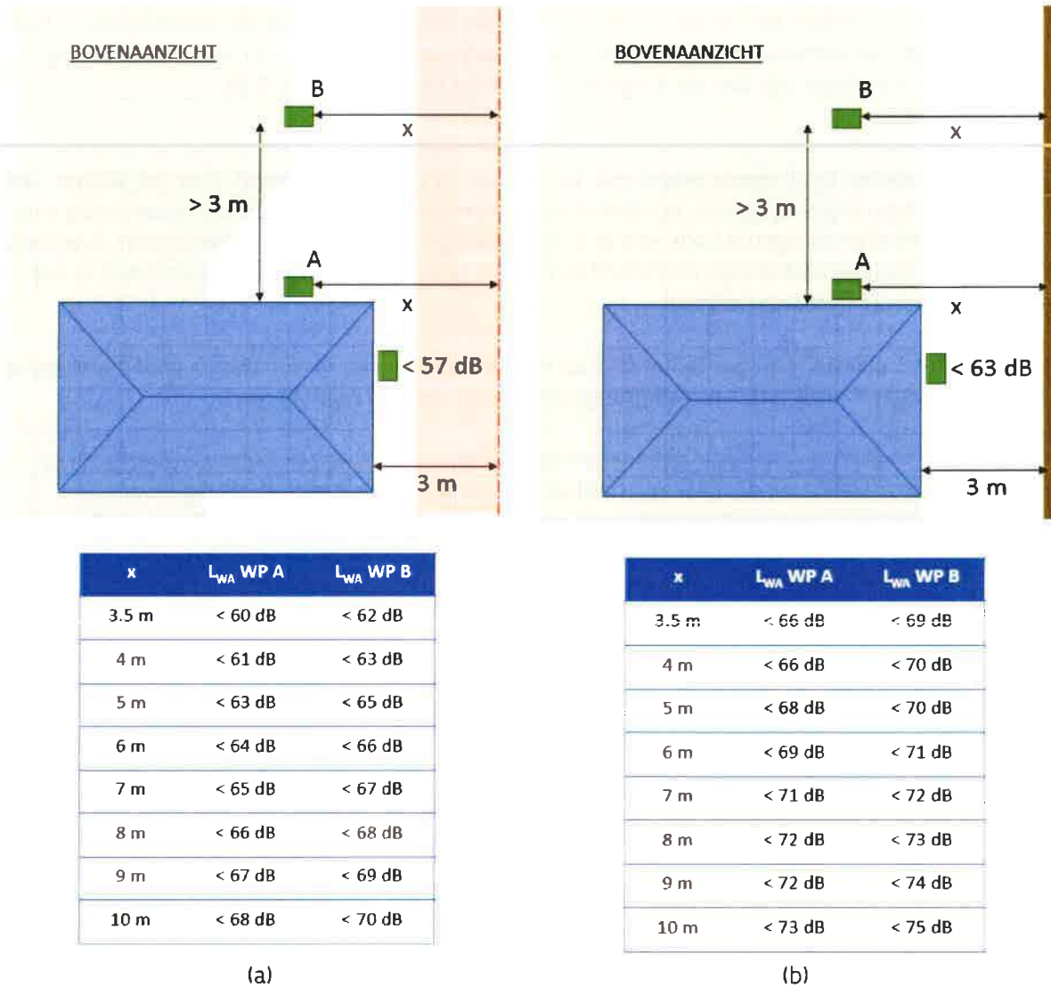
Figuur 10: Maximale geluidsvermogeniveaus van de buitenunit voor diverse posities in de tuin (positie A en B) om te voldoen aan de vooropgestelde geluidsvoorwaarde van 45 dB(A) L_{Aeq, \text{min}} overdag ter hoogte van de perceelsgrens. x is de kleinste afstand tot de dichtstbijzijnde perceelsgrens, in dit voorbeeld is hiervoor de perceelsgrens rechts gekozen. De geluidsbron wordt verondersteld op 0,75 m (2/3 van de hoogte van de unit) en de geluidsdruk werd geëvalueerd op de perceelsgrens op 1,5 m hoogte. In situatie (a) zijn geen afsluitingen tussen de tuinen die een voldoende massa hebben om te zorgen voor afscherming. In situatie (b) is er een volledig gesloten afsluiting met hoogte 1,8 m en oppervlaktemassa \geq 10 \text{ kg/m}^2 aanwezig over de volledige lengte van de perceelsgrens. Daarnaast wordt voor de 2 situaties ook het maximale geluidsvermogen weergegeven voor een buitenunit geplaatst bij de zijgevel op 3 m van de perceelsgrens. Merk op dat in bovenstaande figuur links geen perceelsgrens ingetekend is. Men moet de afstanden in bovenstaande figuur dus ook steeds nagaan voor de linkerzijde (gespiegeld). De groene arcering loopt in werkelijkheid niet door tot aan de linkerperceelsgrens! Ook daar zal een rode en witte zone aanwezig zijn.
