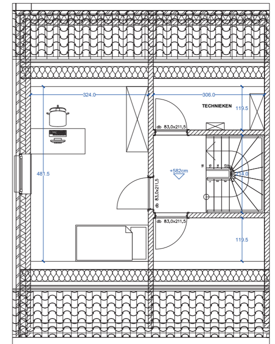
Verdieping +2
