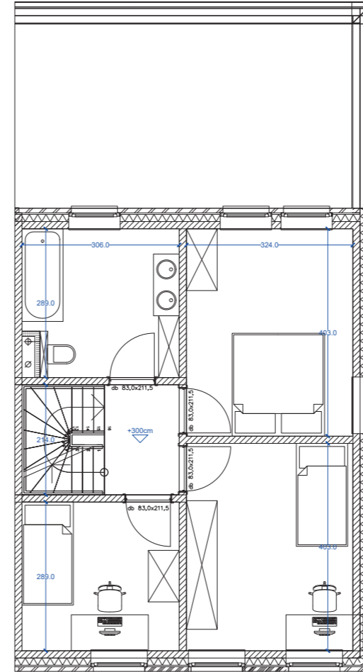
Verdieping +1
