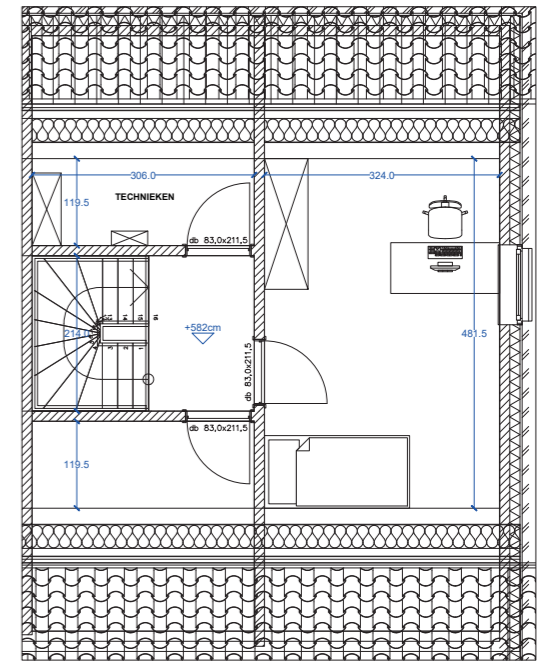
Verdieping +2
