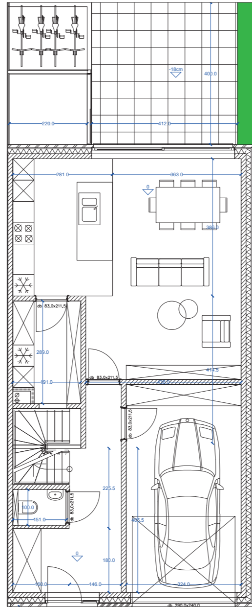
Verdieping +0
