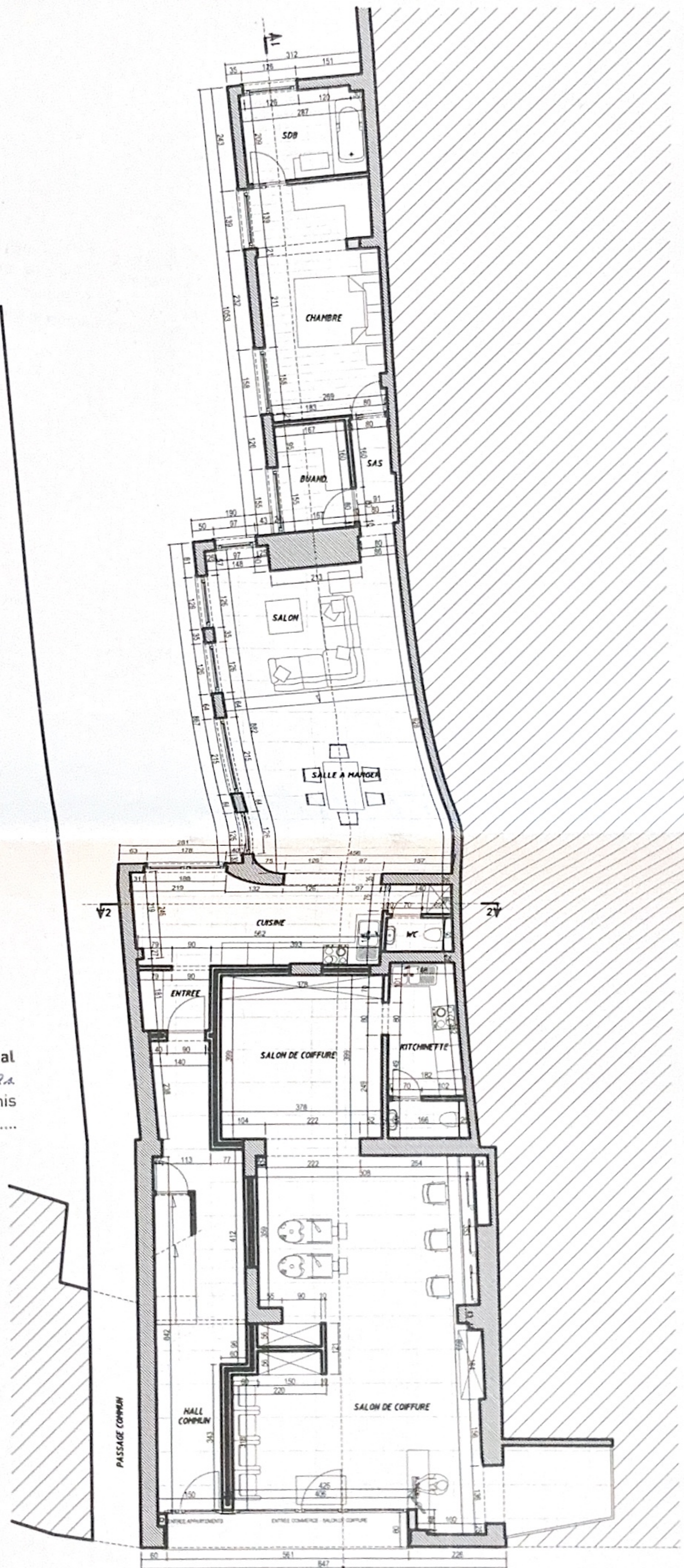
REZ-DE-CHAUSSEE PROJETE ech.: 1/100
