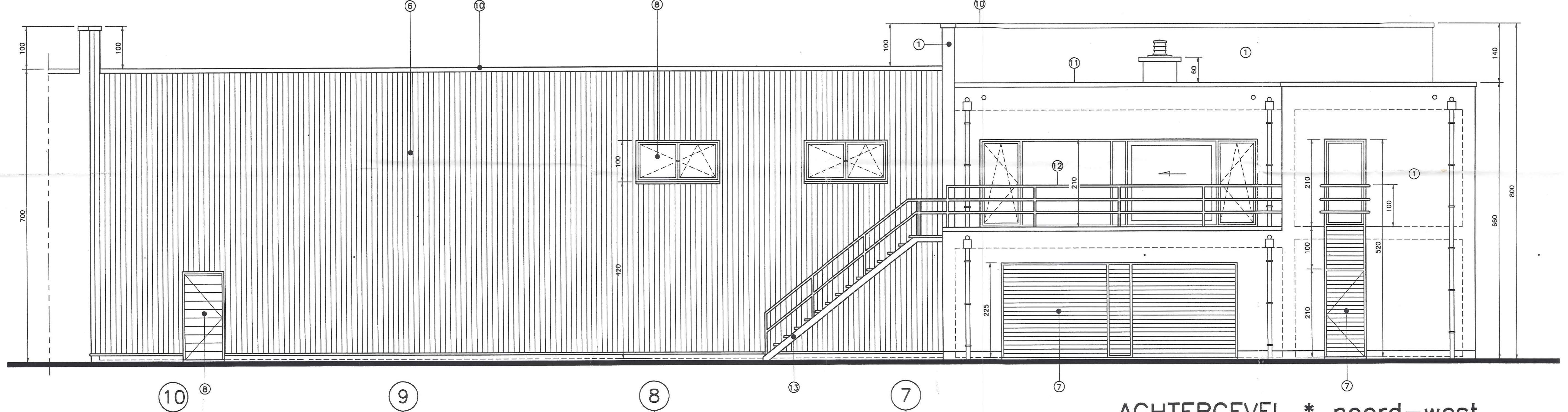
ACHTERGEVEL * noord-west
