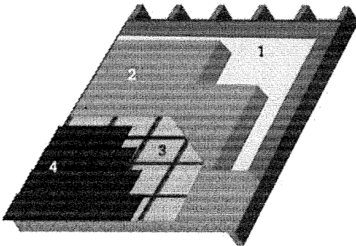
1. Dampscherm | 2. Isolatie | 3. Onderdak | 4. Dakbedekking
