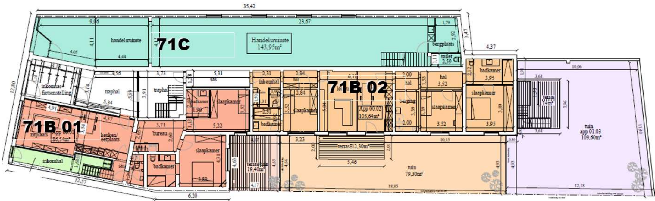
Gelijkvloerse verdieping
