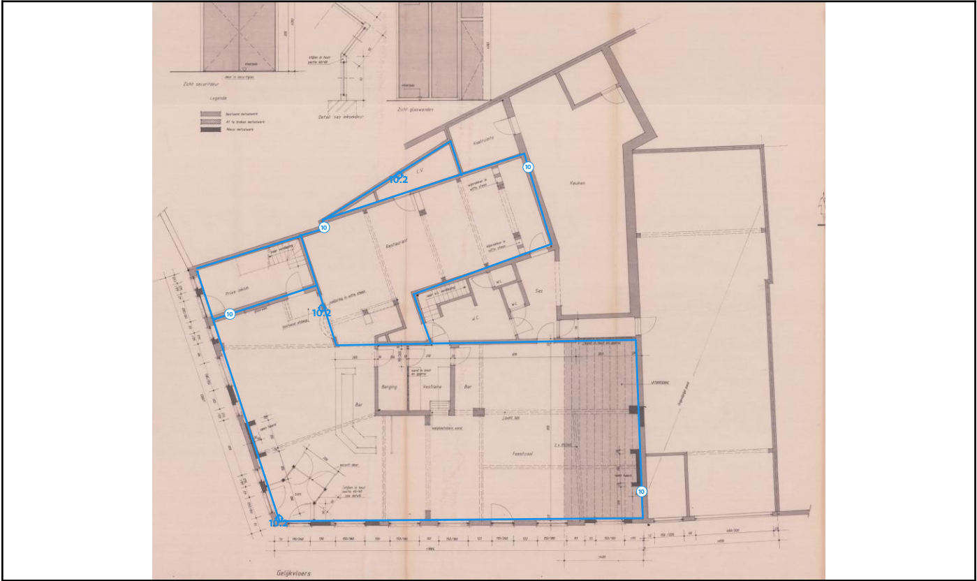
Legende van plan 1.5: Gelijkvloers - detail pleisterwerk
