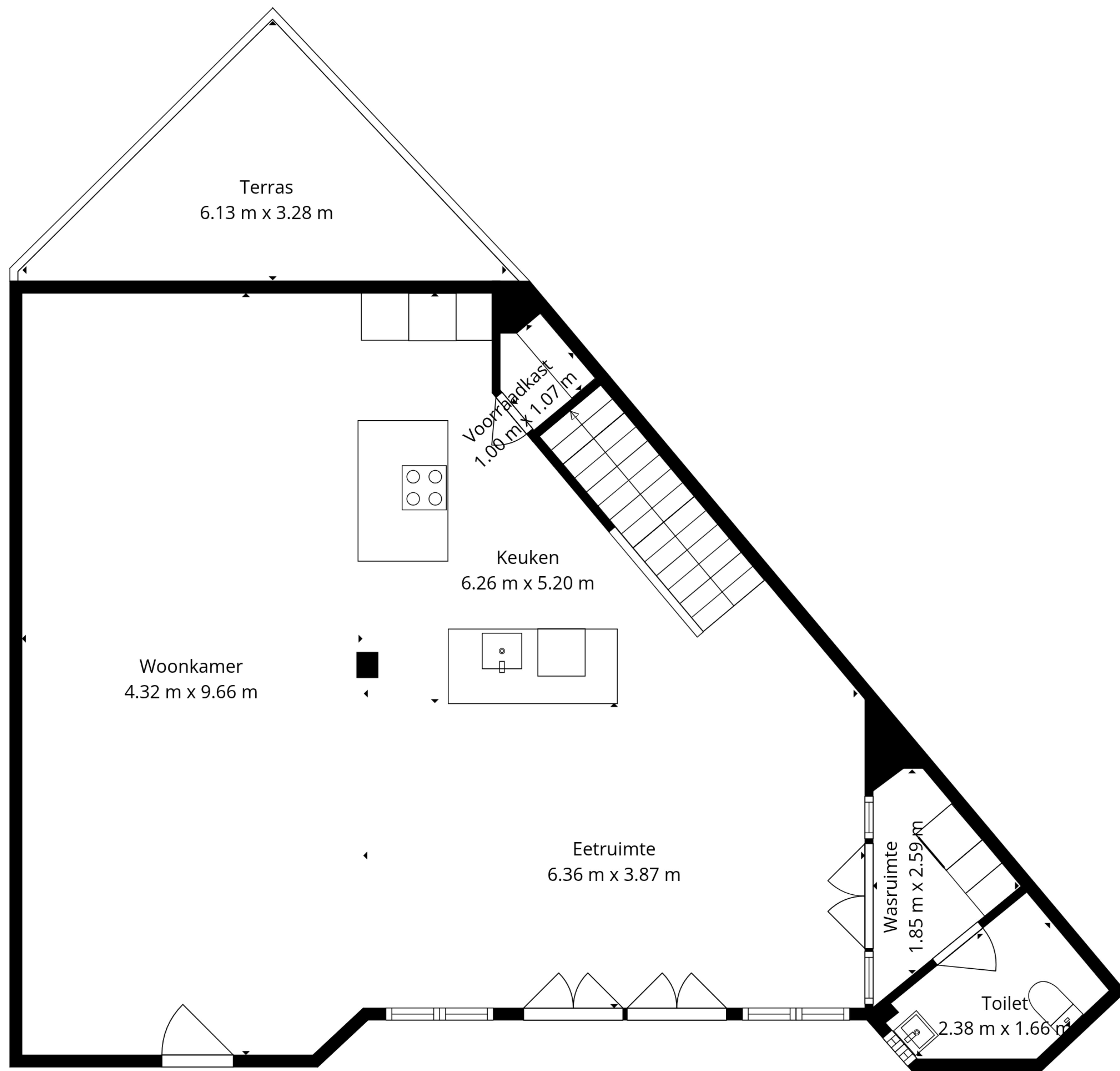
1e Verdieping
