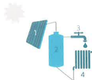
1 Zonnecollector | 2 Opslagvat voor warm water | 3 Sanitair (bijv. badstoft) | 4 Radiator (voor ruimteverwarming)
