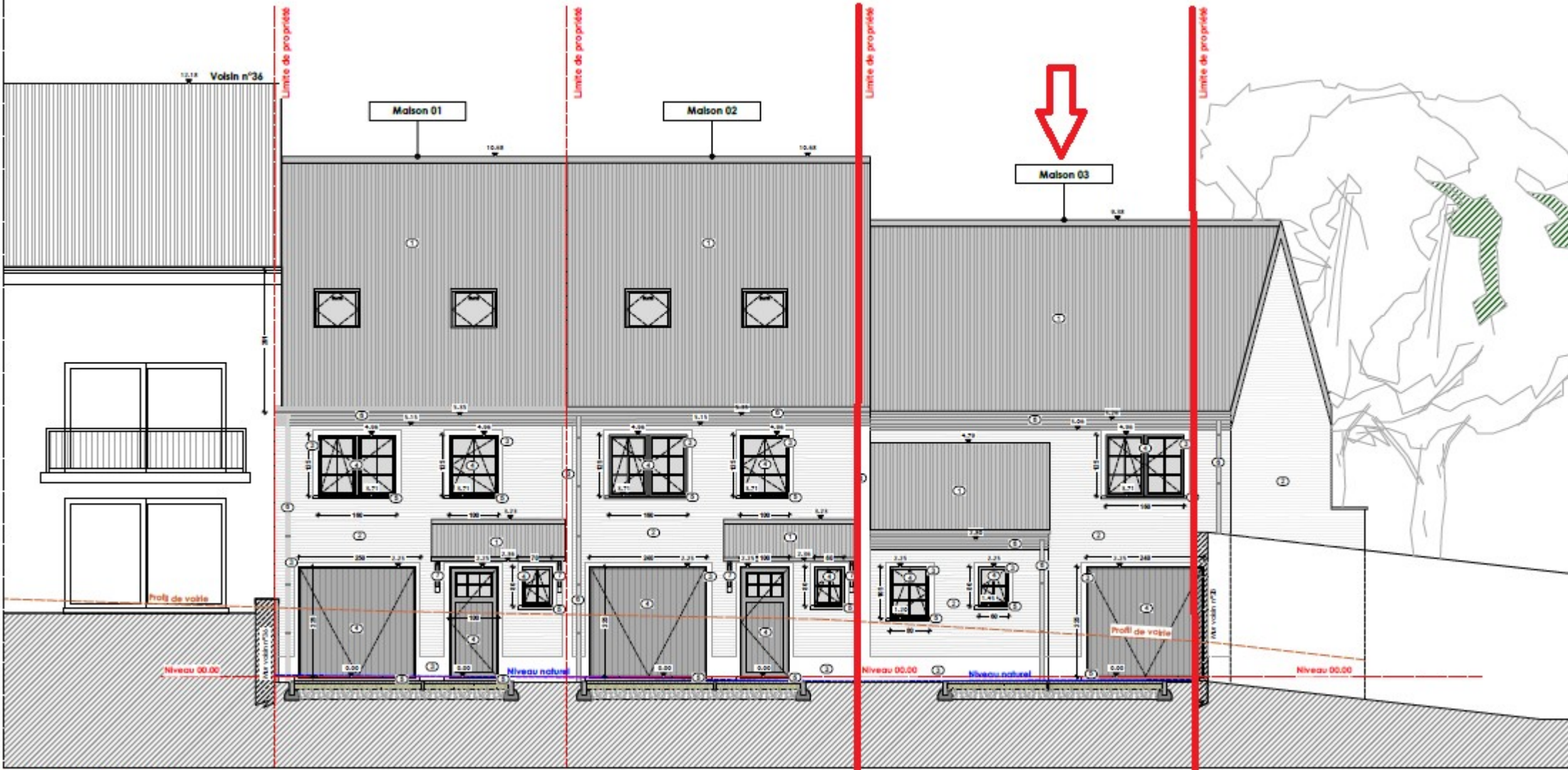
Elevation SUD (côté rue)
