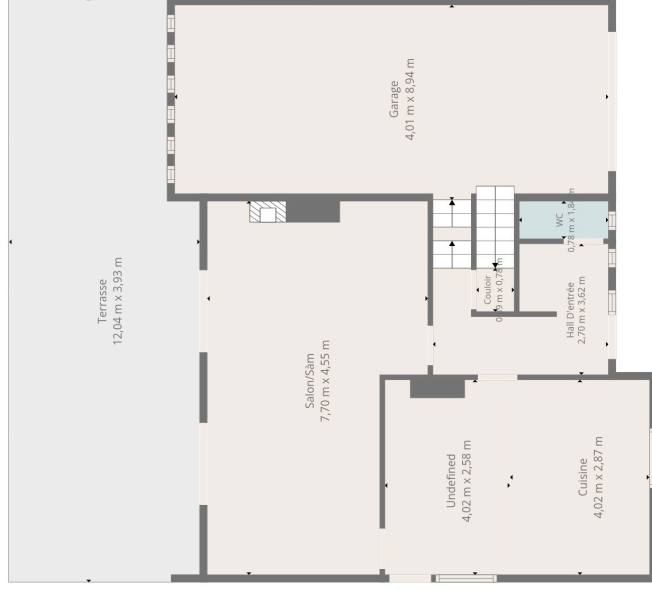
Rez-de-chaussée
