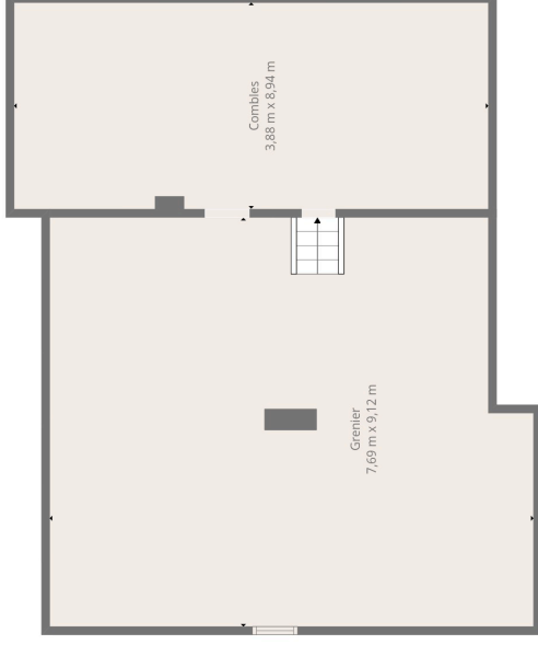
3ème Étage
