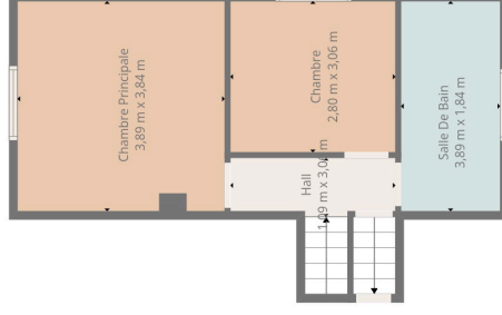
1er Étage
