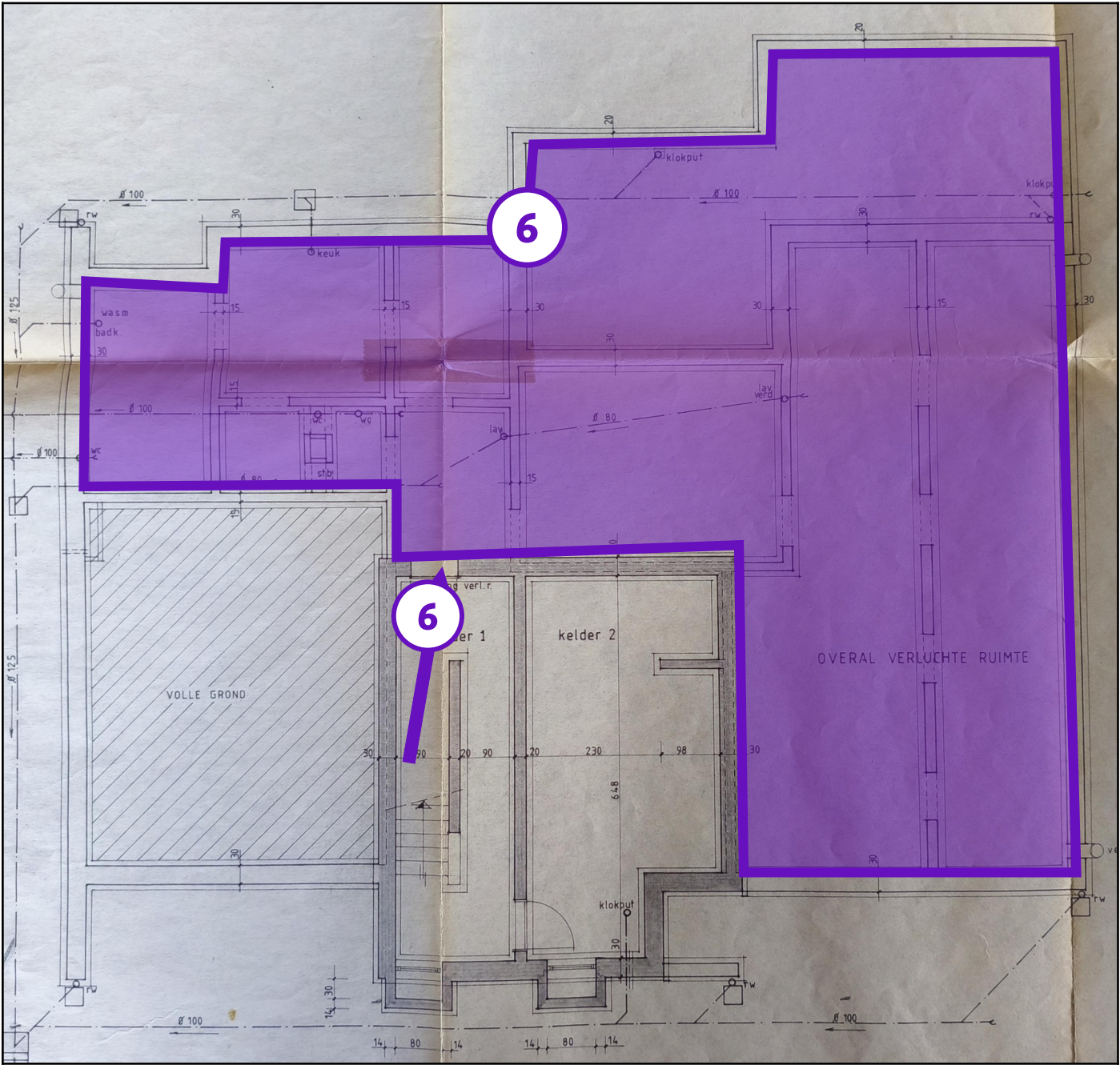
Legende van plan 1.4: Fundering - kelder
