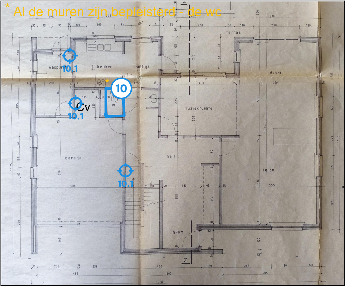
Legende van plan 1.9: Gelijkvloers
