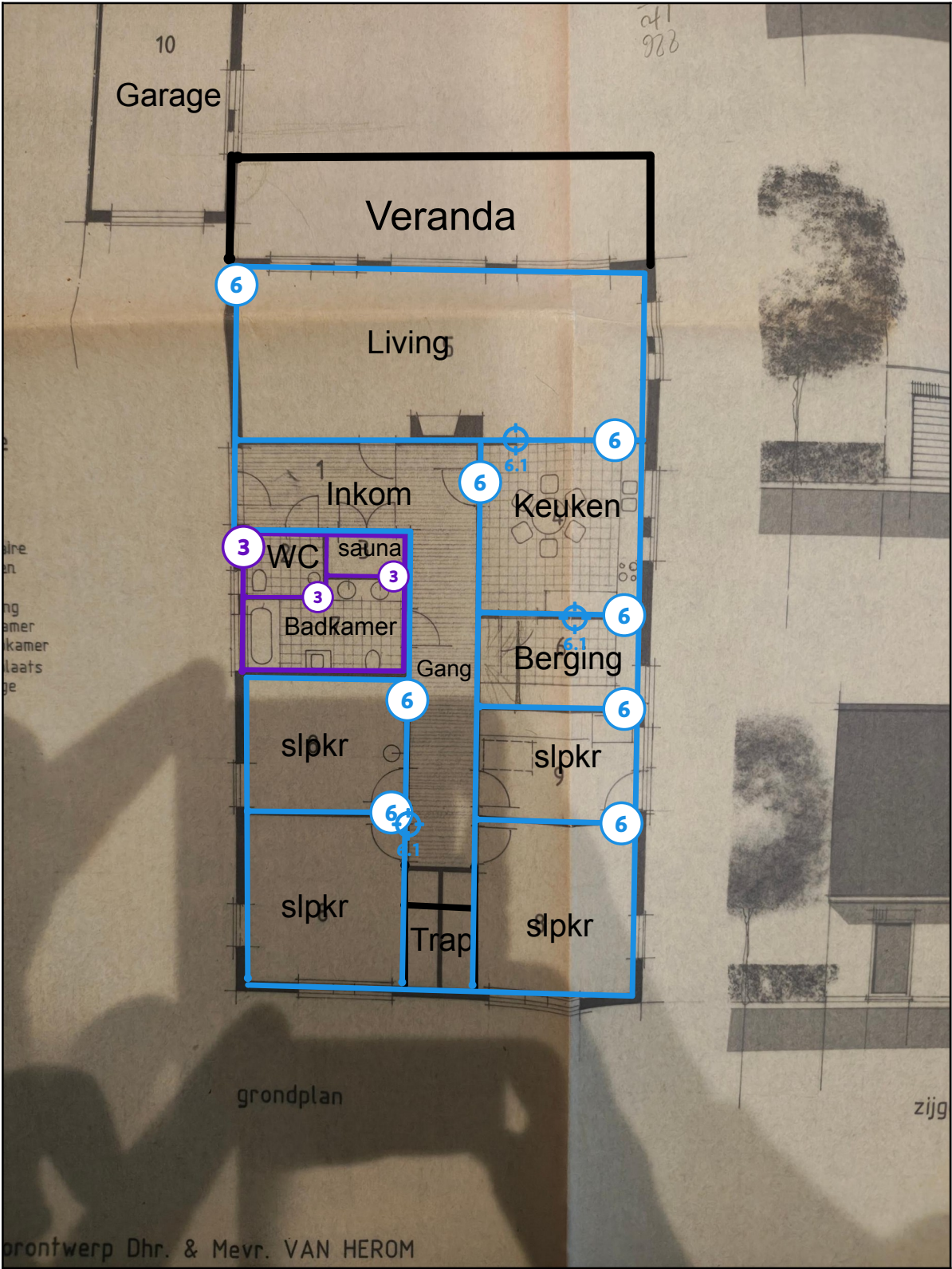
Legende van plan 1.4: Gelijkvloers (muren)
