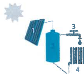
1 Zonnecollector 2 Opslagvat 3 Tap 4 Verbruiker (radiator)
