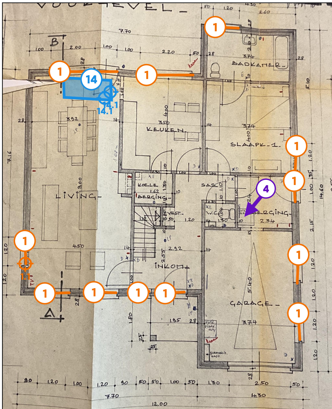
Legende van plan 1.5: GLV: kruipruimte / kit / cementering
