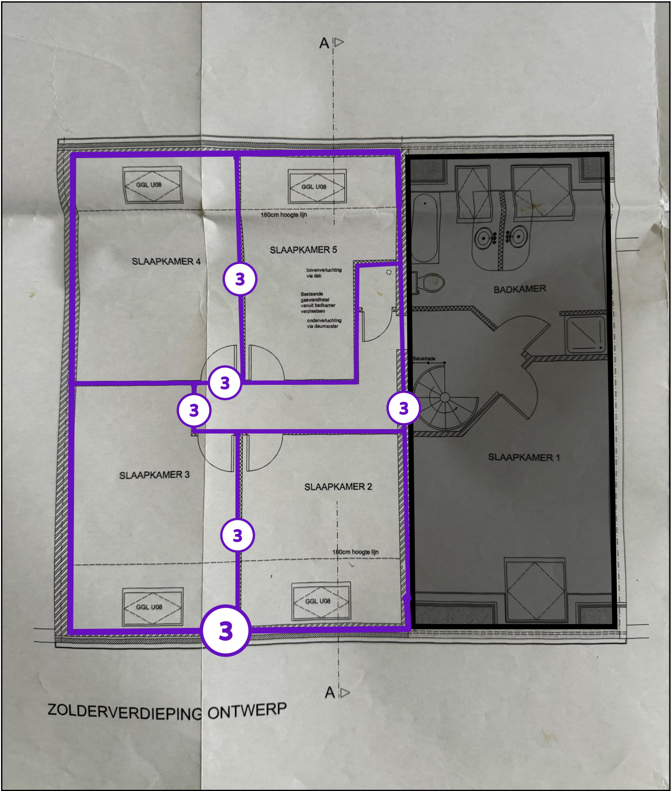
Legende van plan 1.5: Tweede verdiep; valse wand
