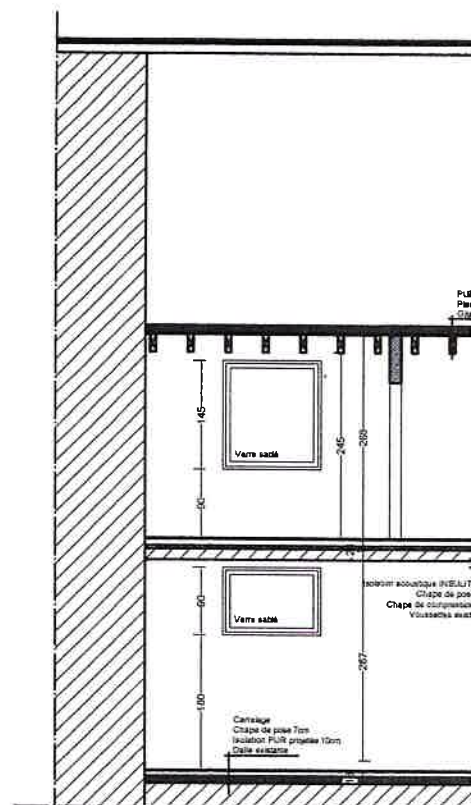
Coupe BB éch. : 1/100
