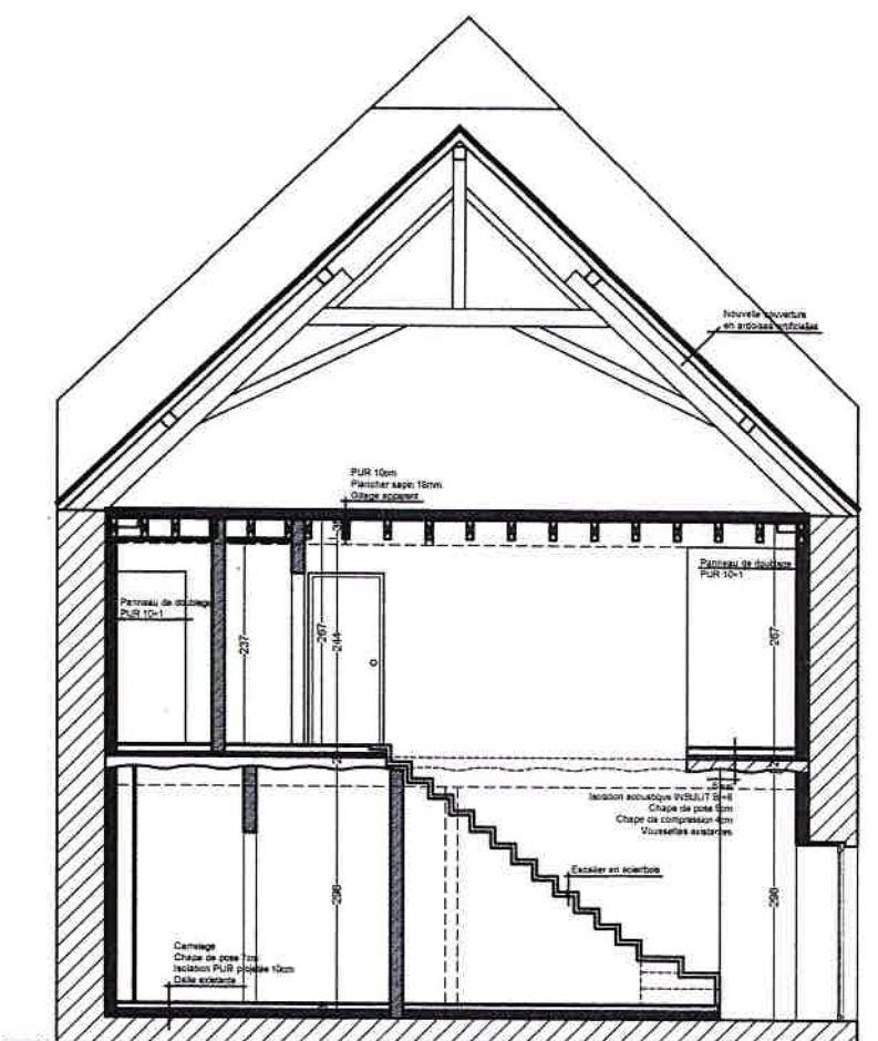
Coupe AA éch. : 1/100
