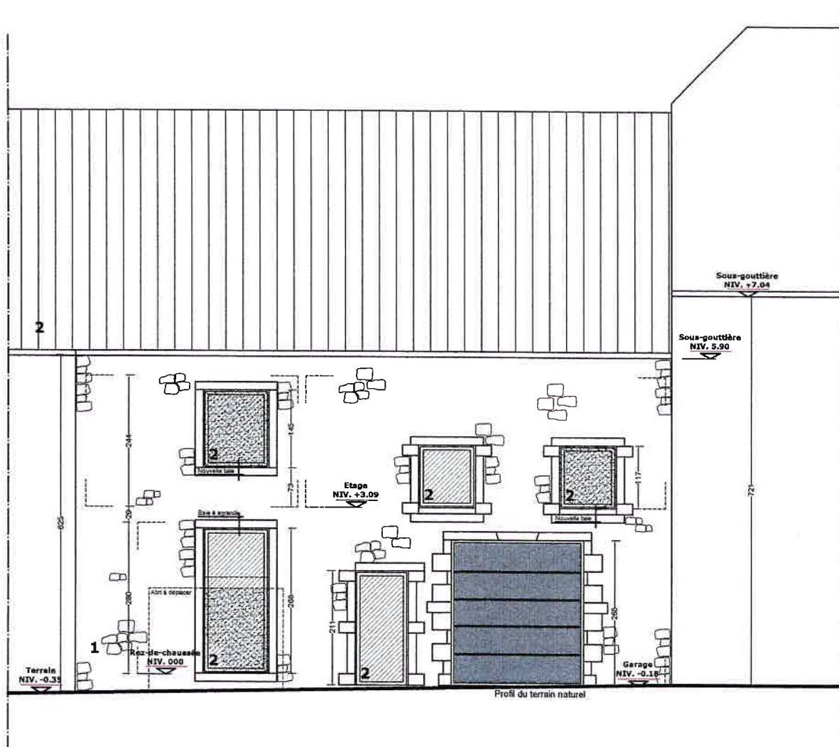
Façade principale éch. : 1/100
