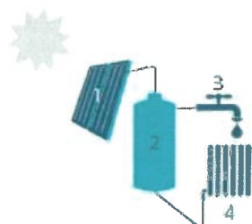
1 Zonnecollector | 2 Opslagvat zonnecoö | 3 Sanitair warm water | 4 Afgifte-element voor ruimteverwarming (optioneel)
