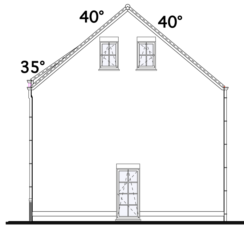
RECHTER GEVEL
