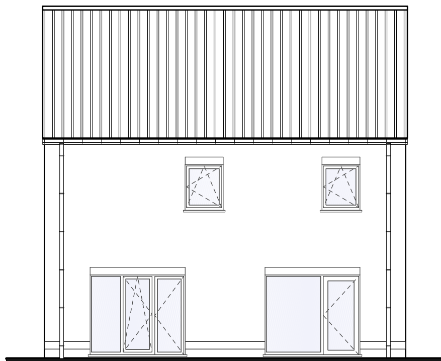
ACHTERGEVEL
