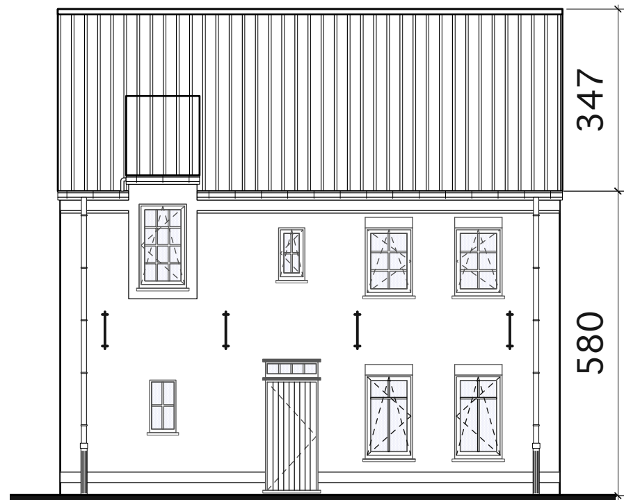
VOORGEVEL
