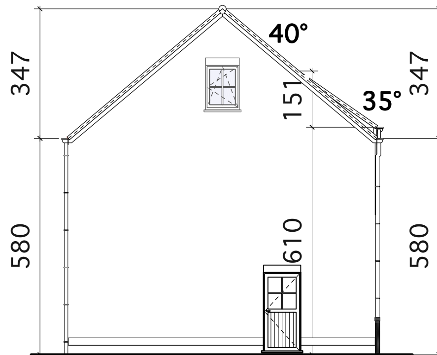
LINKER GEVEL
