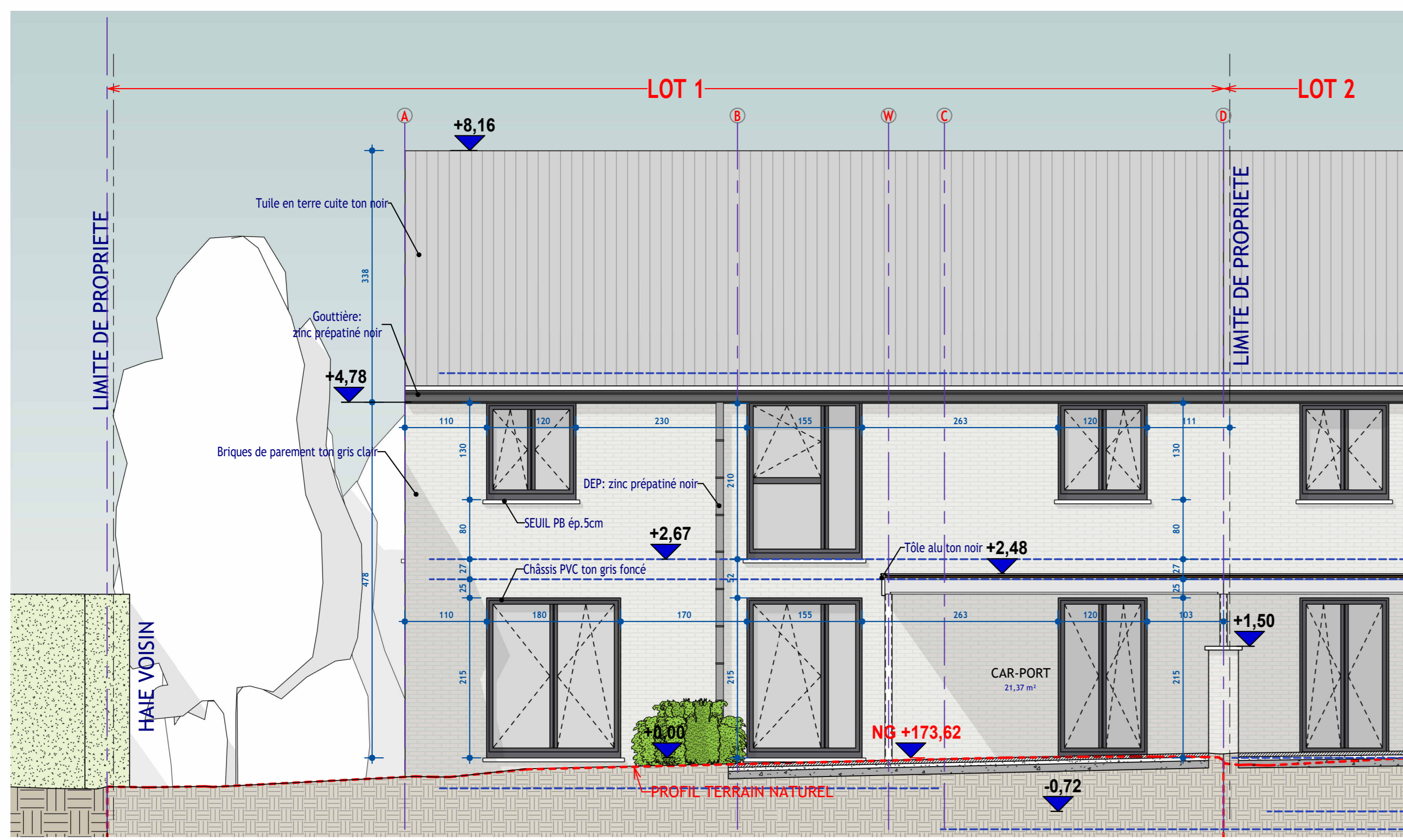
2 LOT 1 - ELEVATION SUD-OUEST Ech : 1 : 50
