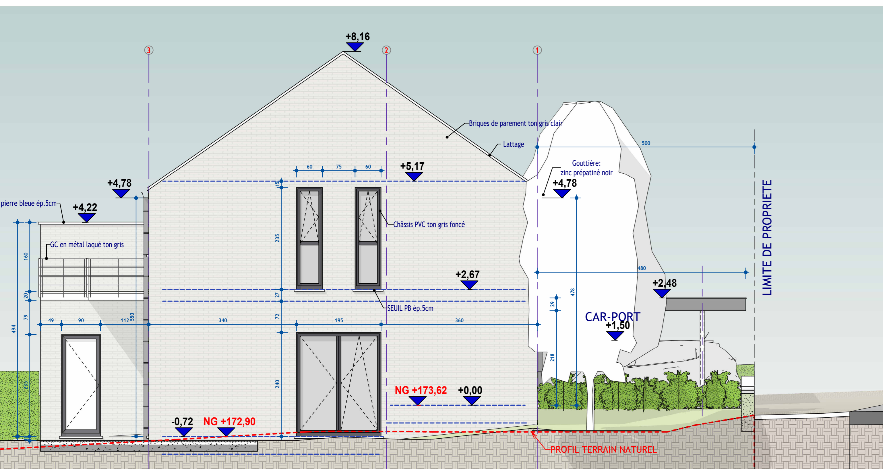
1 LOT 1 - ELEVATION NORD-OUEST Ech : 1 : 50
