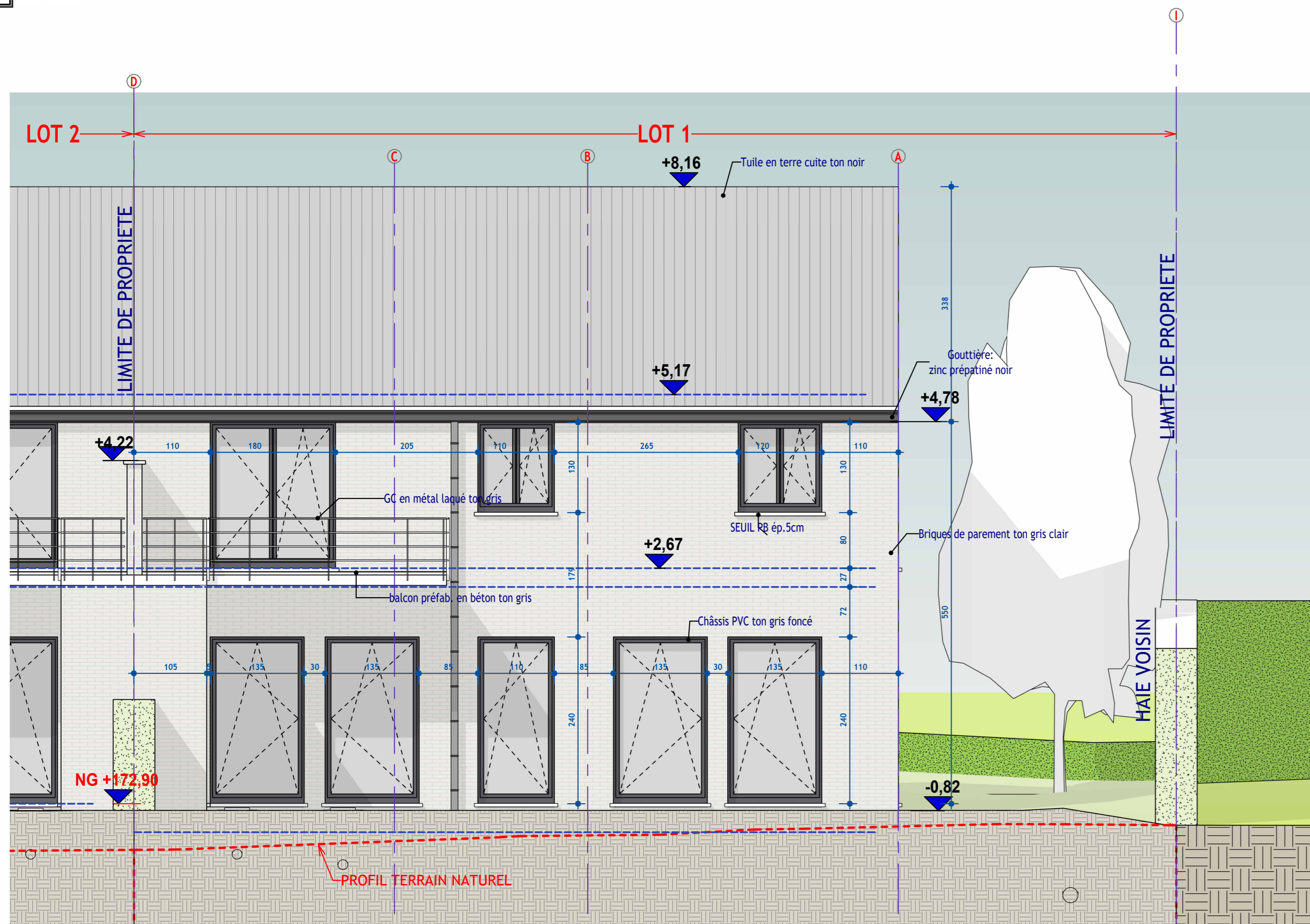
3 LOT 1 - ELEVATION NORD-EST Ech : 1 : 50
