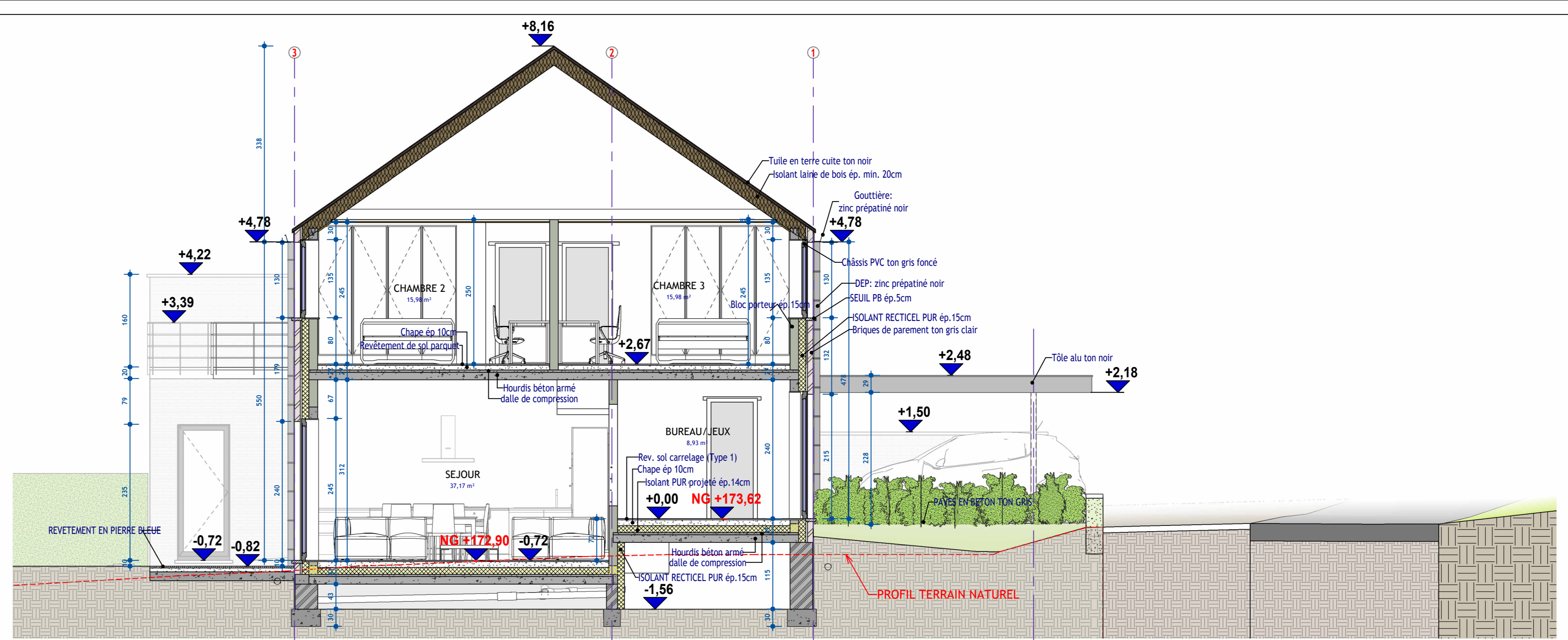
1-A COUPE A-A Ech : 1 : 50
