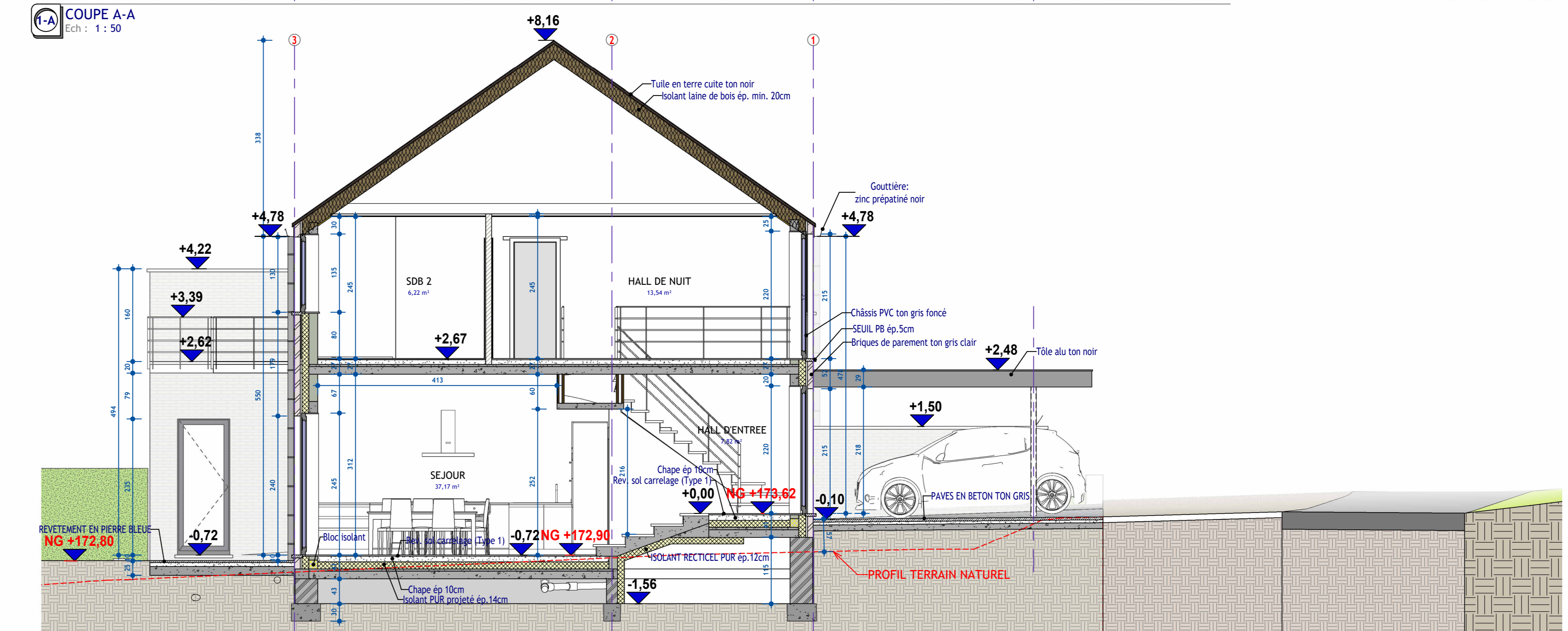
1-B COUPE B-B Ech : 1 : 50
