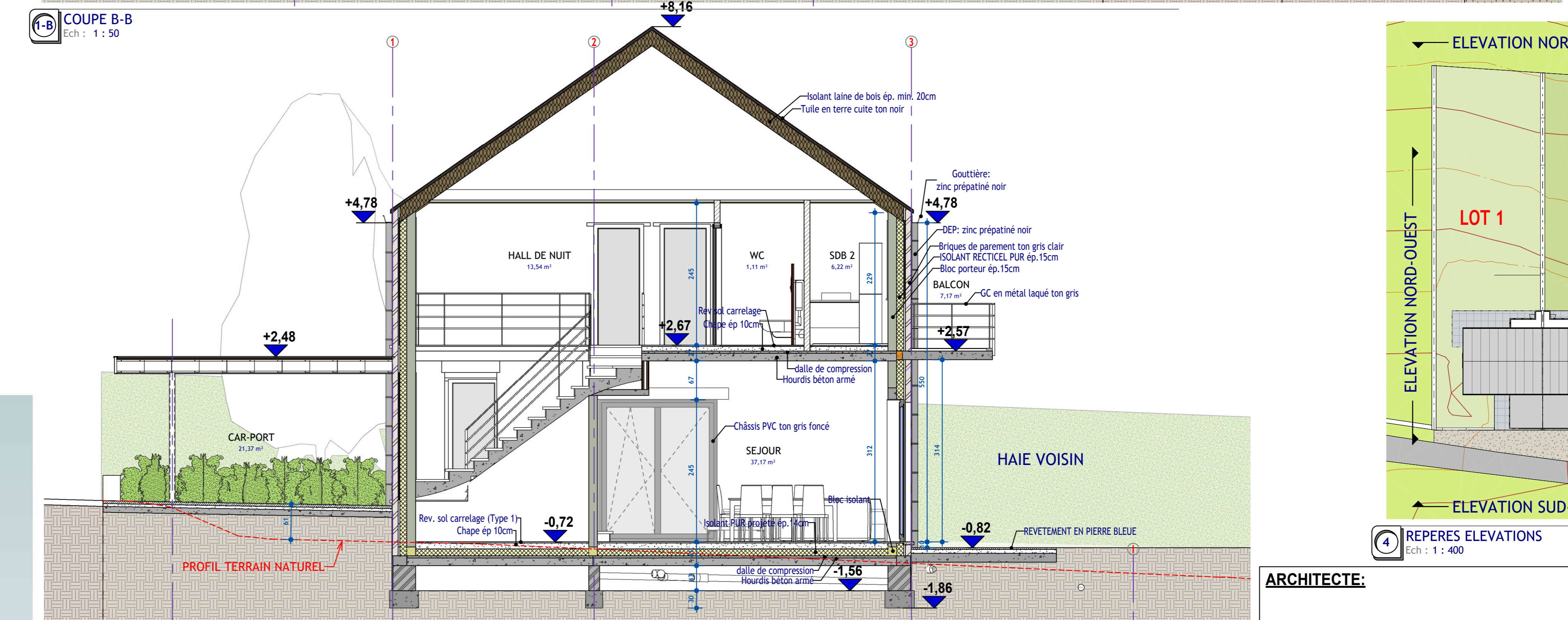
1-C COUPE C-C Ech : 1 : 50
