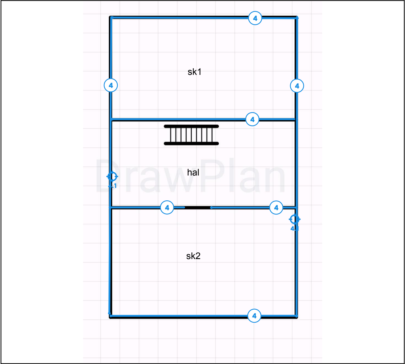
Legende van plan 1.3: 1ste verdiep pleisterwerk muren
