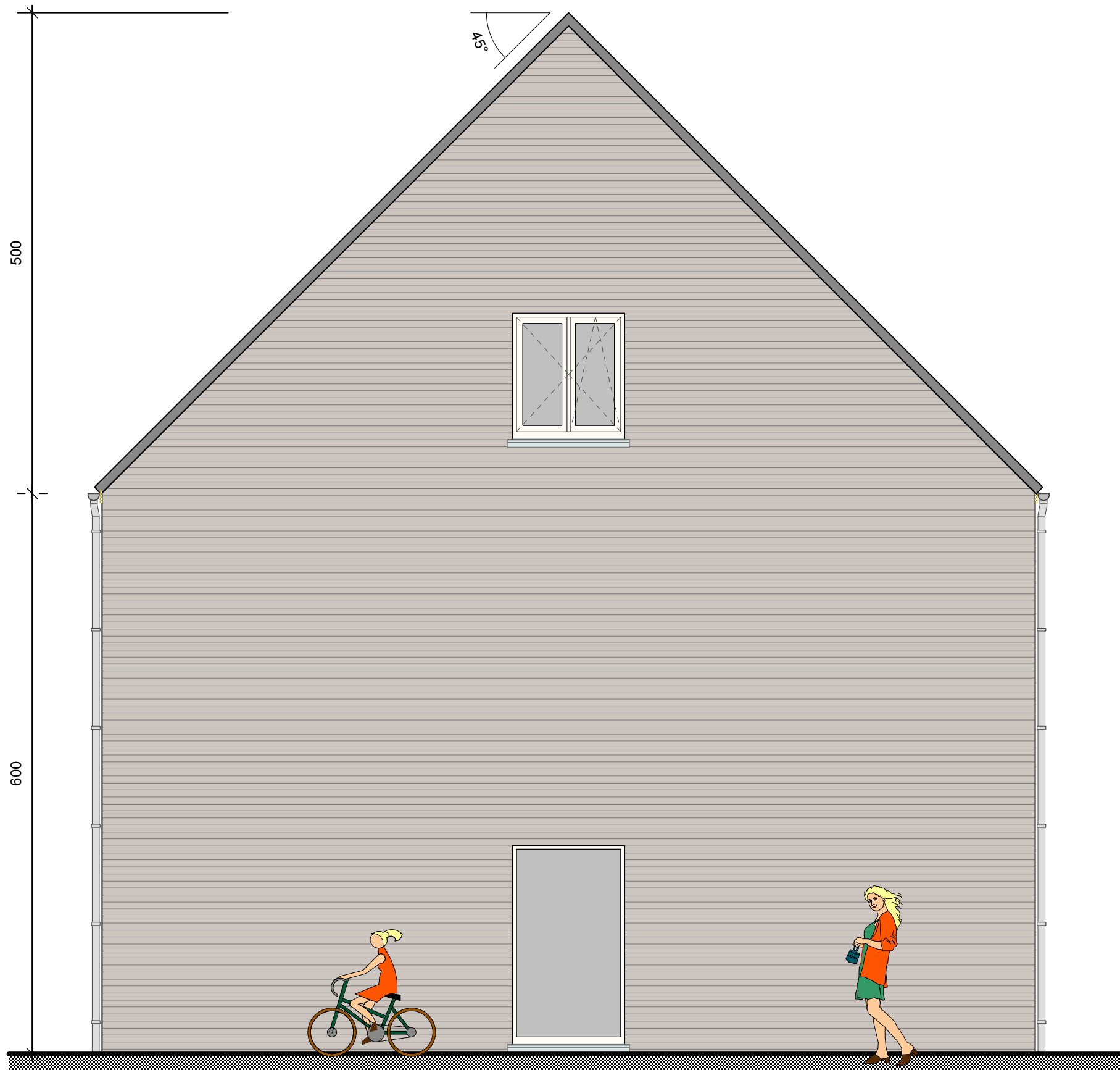
Zijgevel rechts
