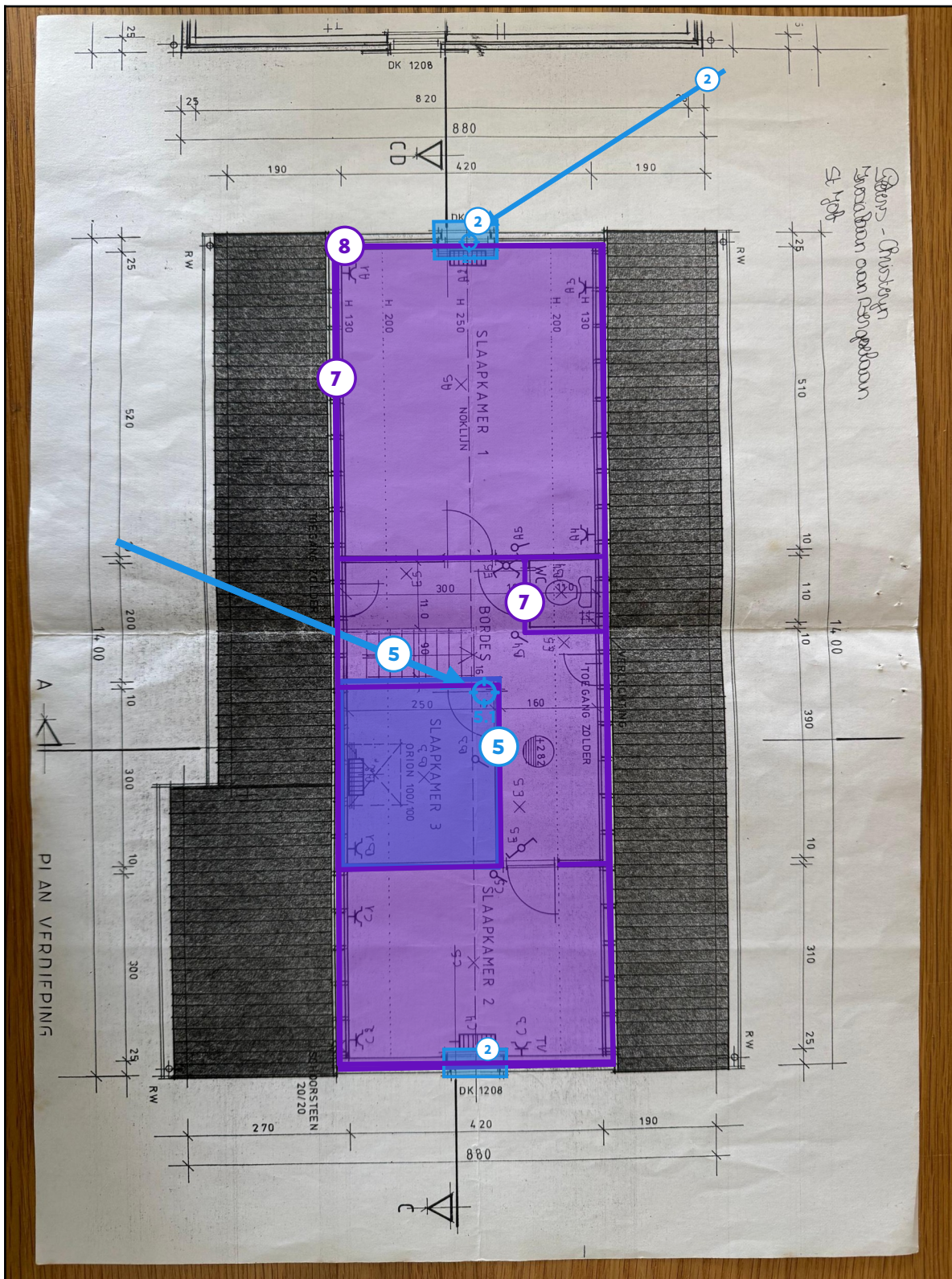
Legende van plan 1.2: Eerste verdieping
