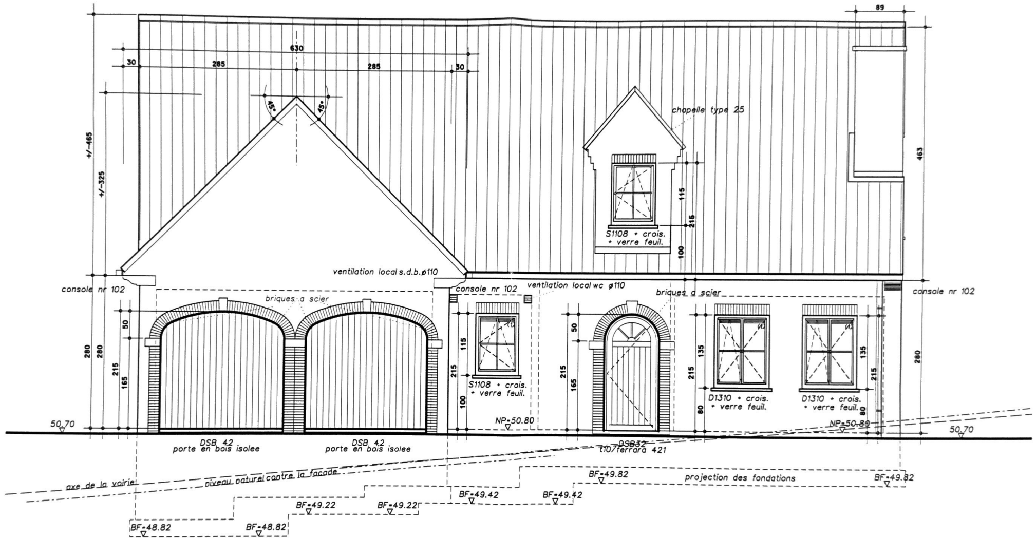
(1) Mécanisme de ventilation incorporé au châssis FACADE PRINCIPALE ech 1/50
