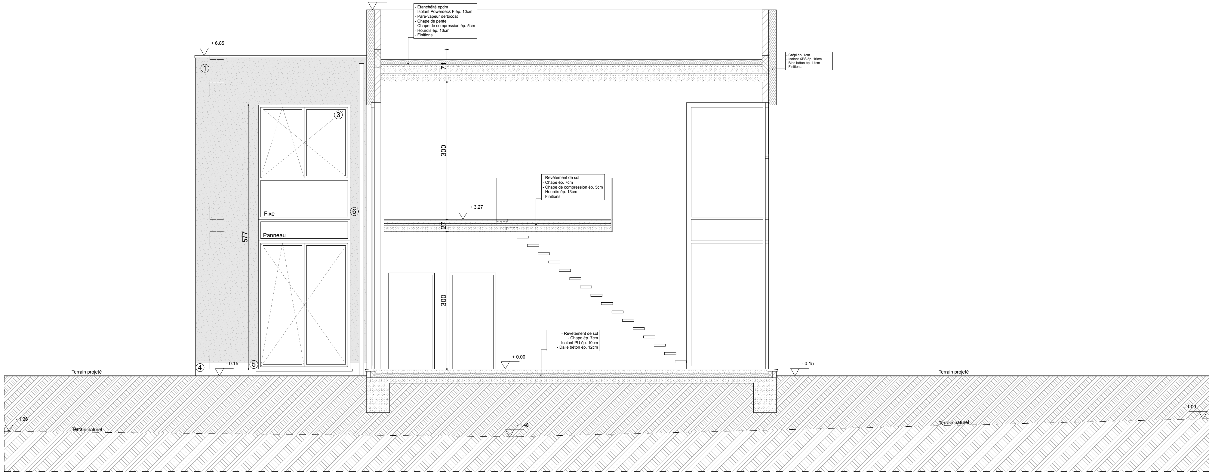
Coupe BB 1/50
