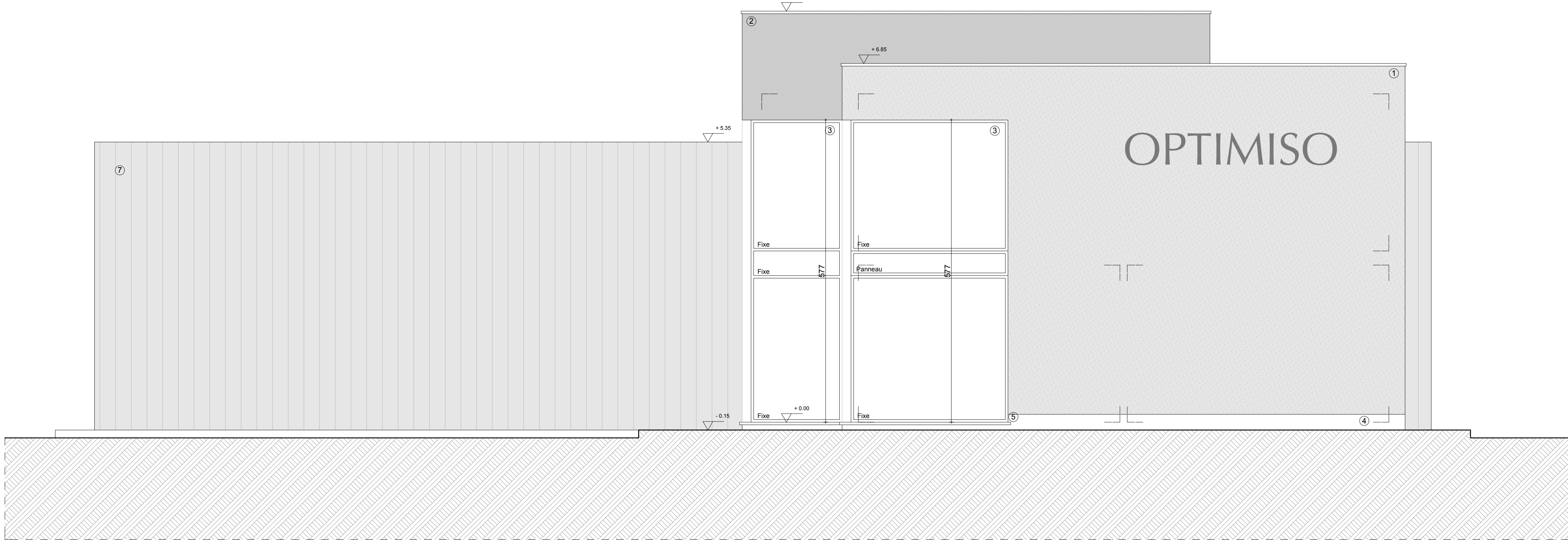
Façade avant 1/50
