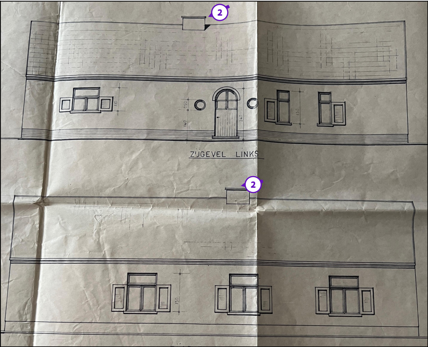
Legende van plan 1.6: Grondplan dak
