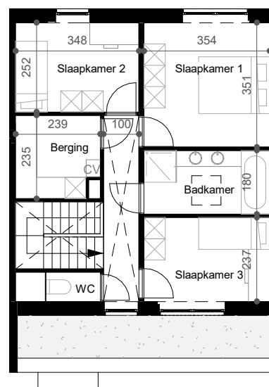
NIVEAU +1 1/150
