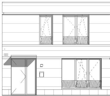
VOORGEVEL 1/150
