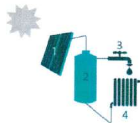
Zonnecollector | 2. Opslagvat zonneboiler | 3. Aantal warm water | 4. Afgifte-element voor ruimteverwarming (optioneel)
