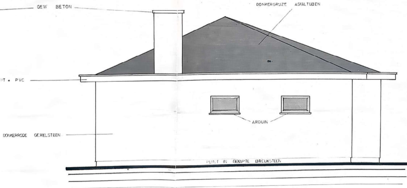
ZIJGEVEL LINKS
