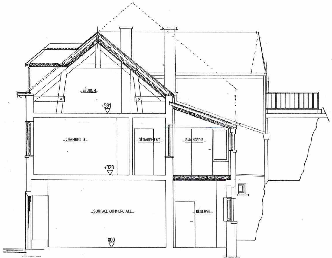
-COUPE A-A.- éch. 1/50 1/100
