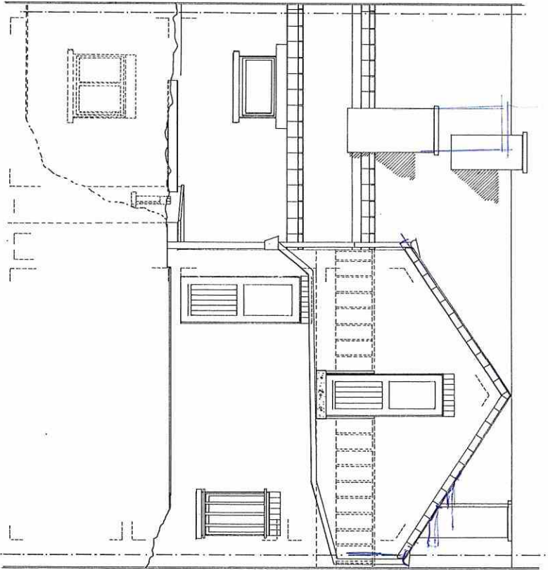
FACADE ARRIÈRE. écl. 1/1000
