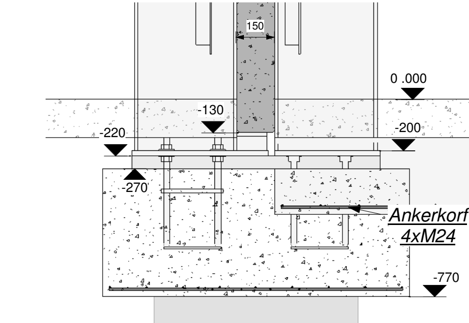
B Voetplaat brandwand 1 : 15
