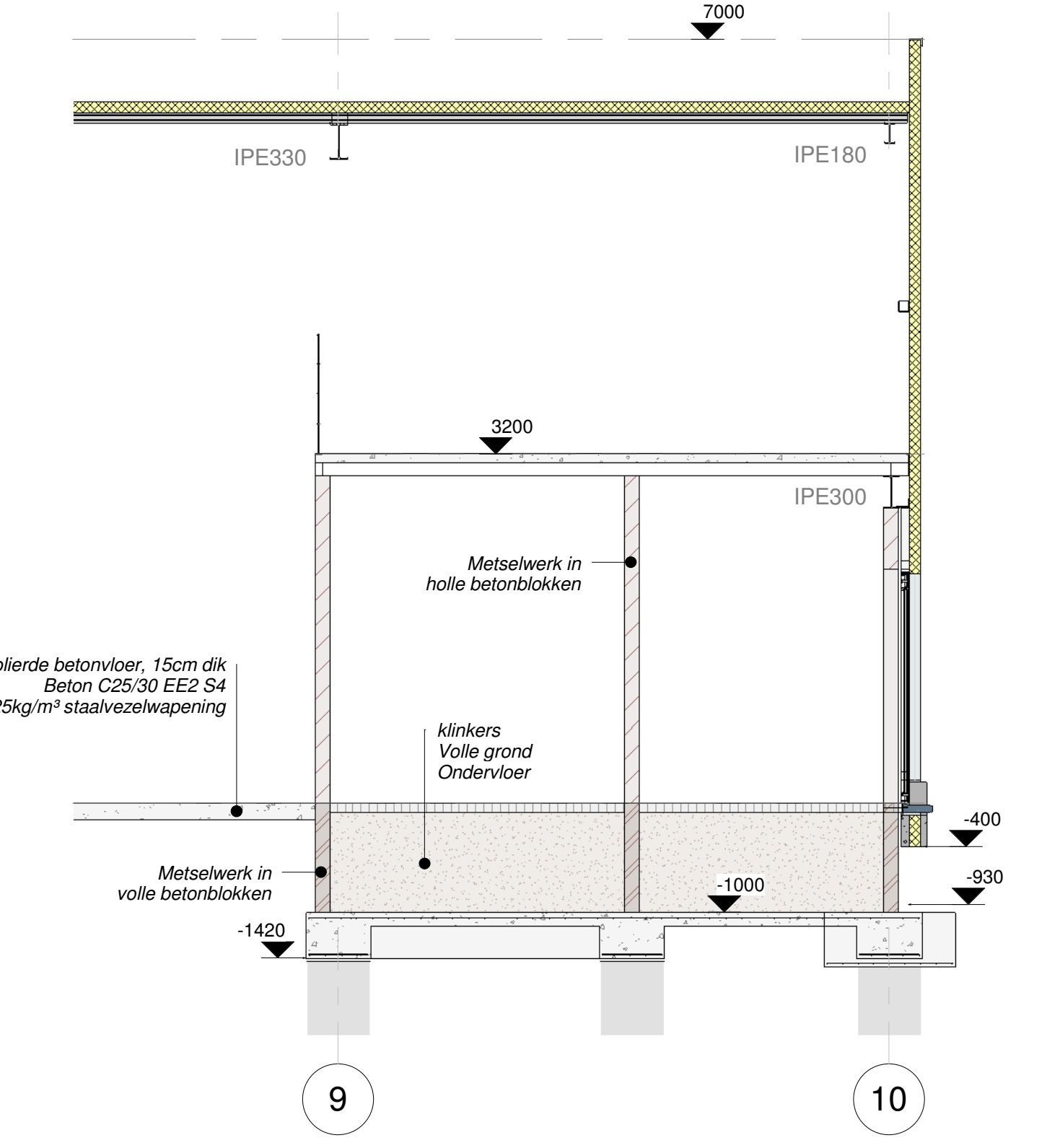
4 Snede technische lokalen 1 : 50
