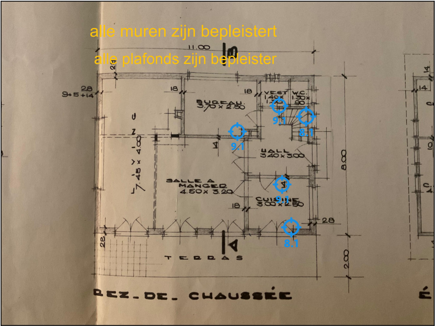
Legende van plan 1.2: Gelijksvloer
