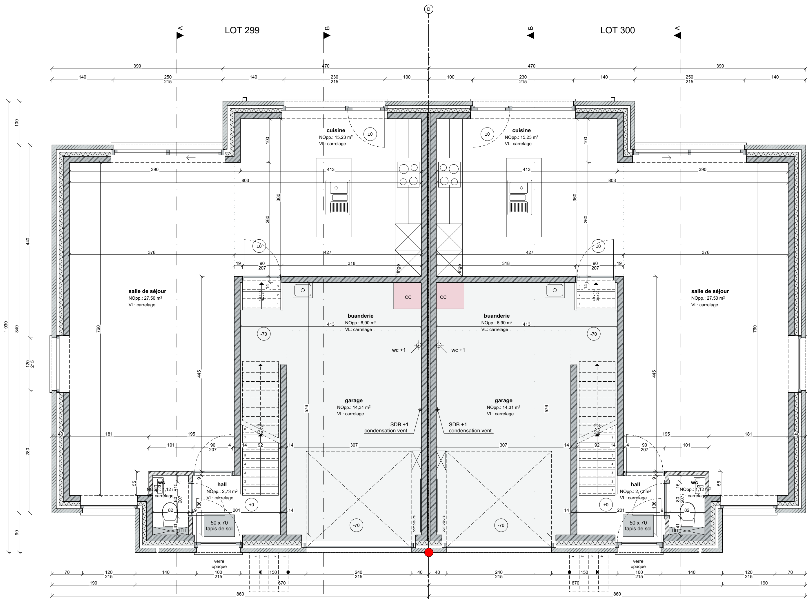
Rez-dechaussée 1:50
