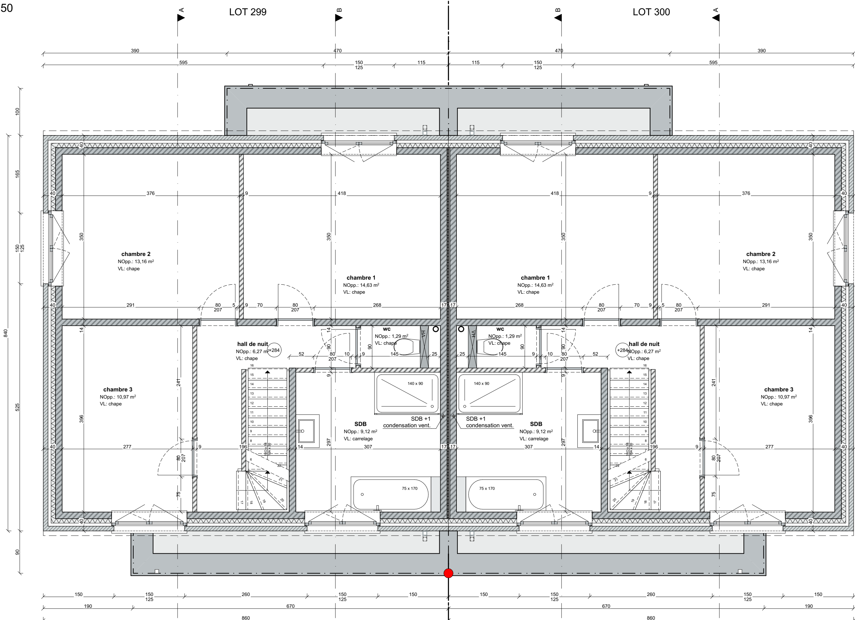
1ère étage 1:50
