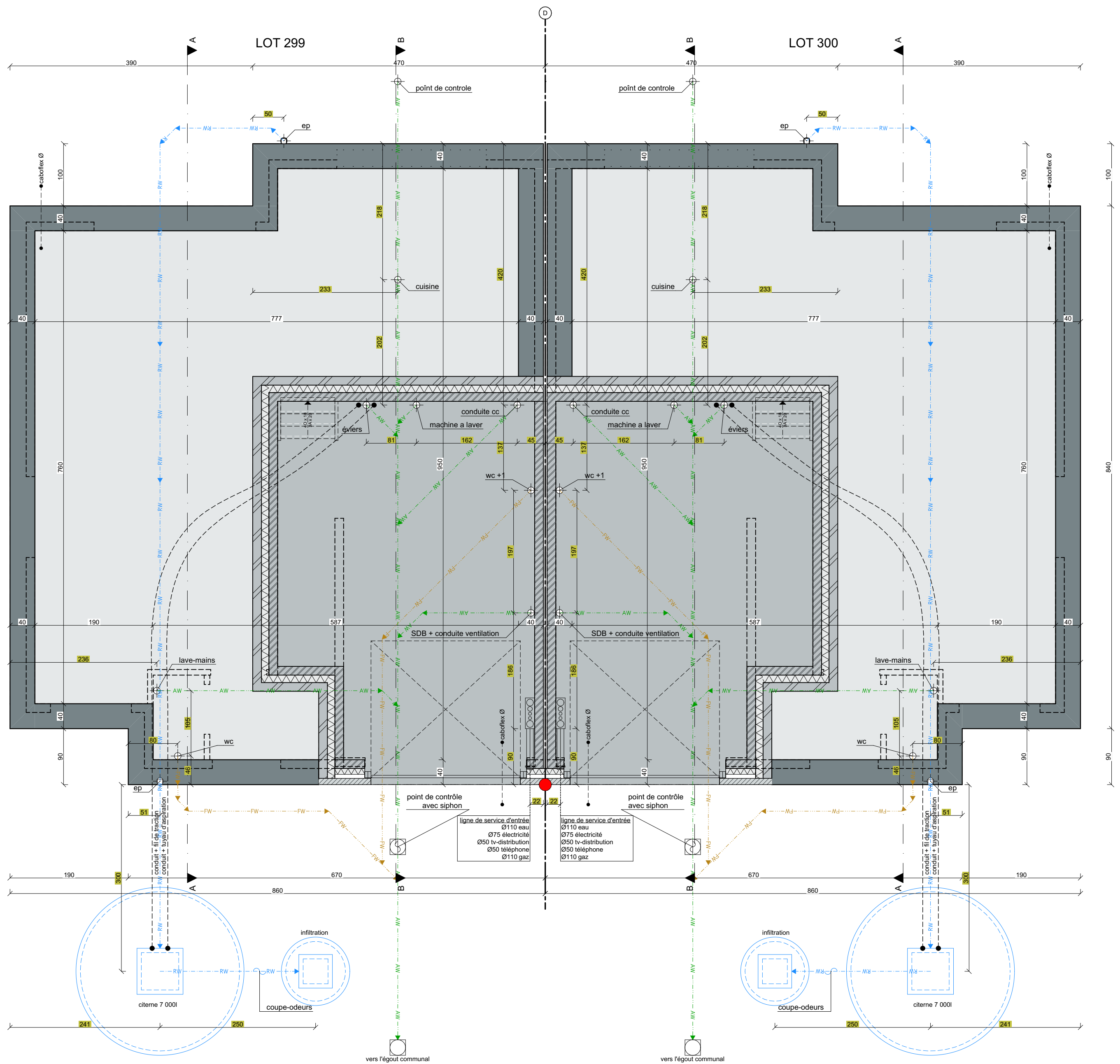
plan des fondations et des égouts 1:50
