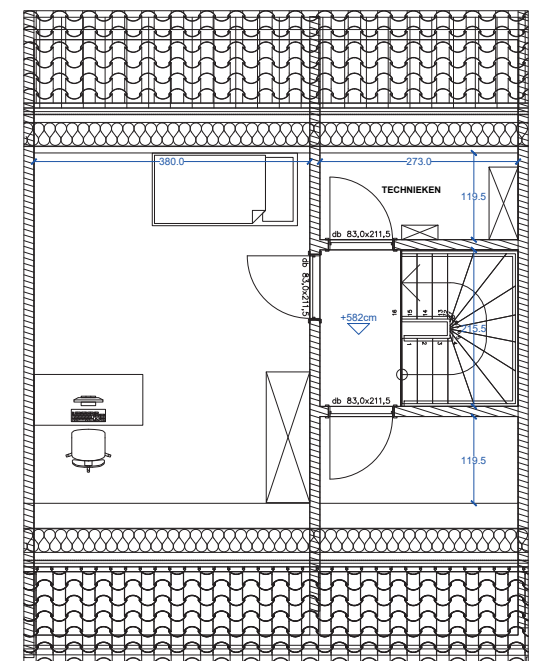
Verdieping +2
