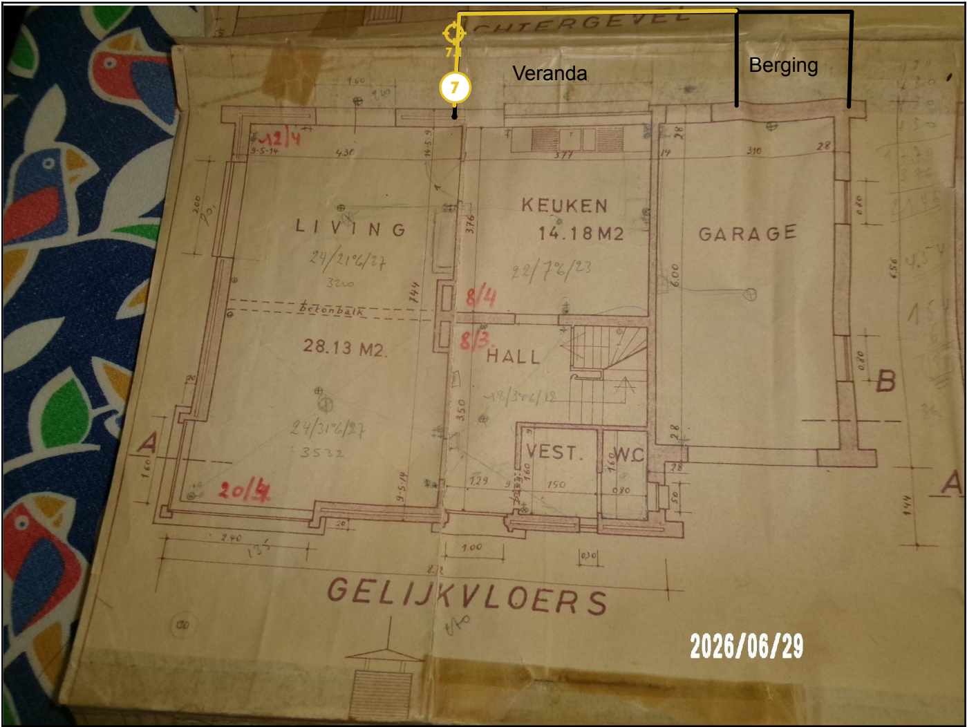
Legende van plan 1.5: Plan gelijkvloers
