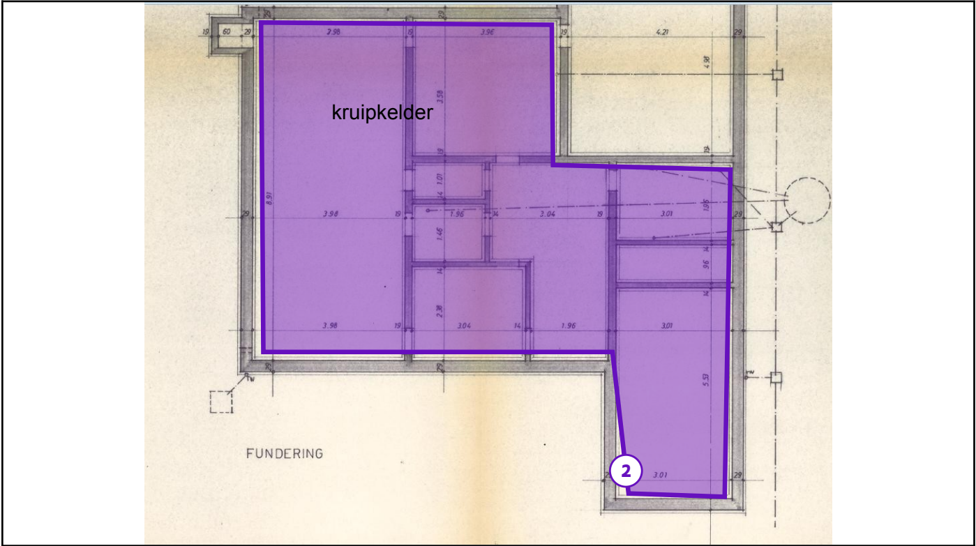
Legende van plan 1.1: Hoofdgebouw plan kruipkelder
