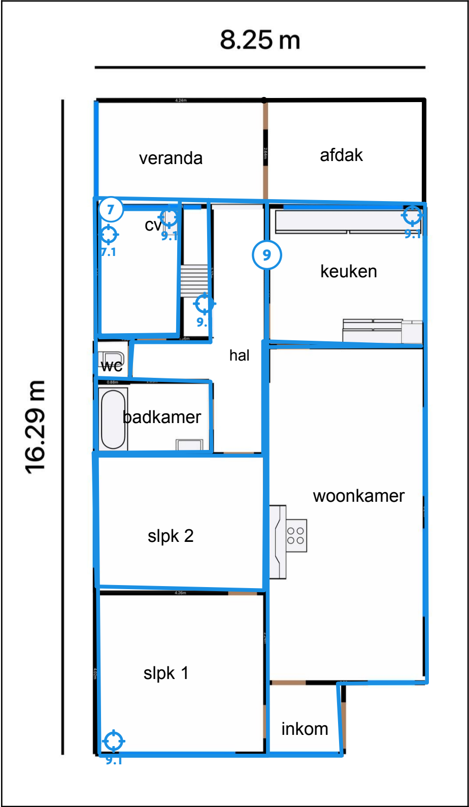
Legende van plan 1.3: Gelijkvloers (wanden)
