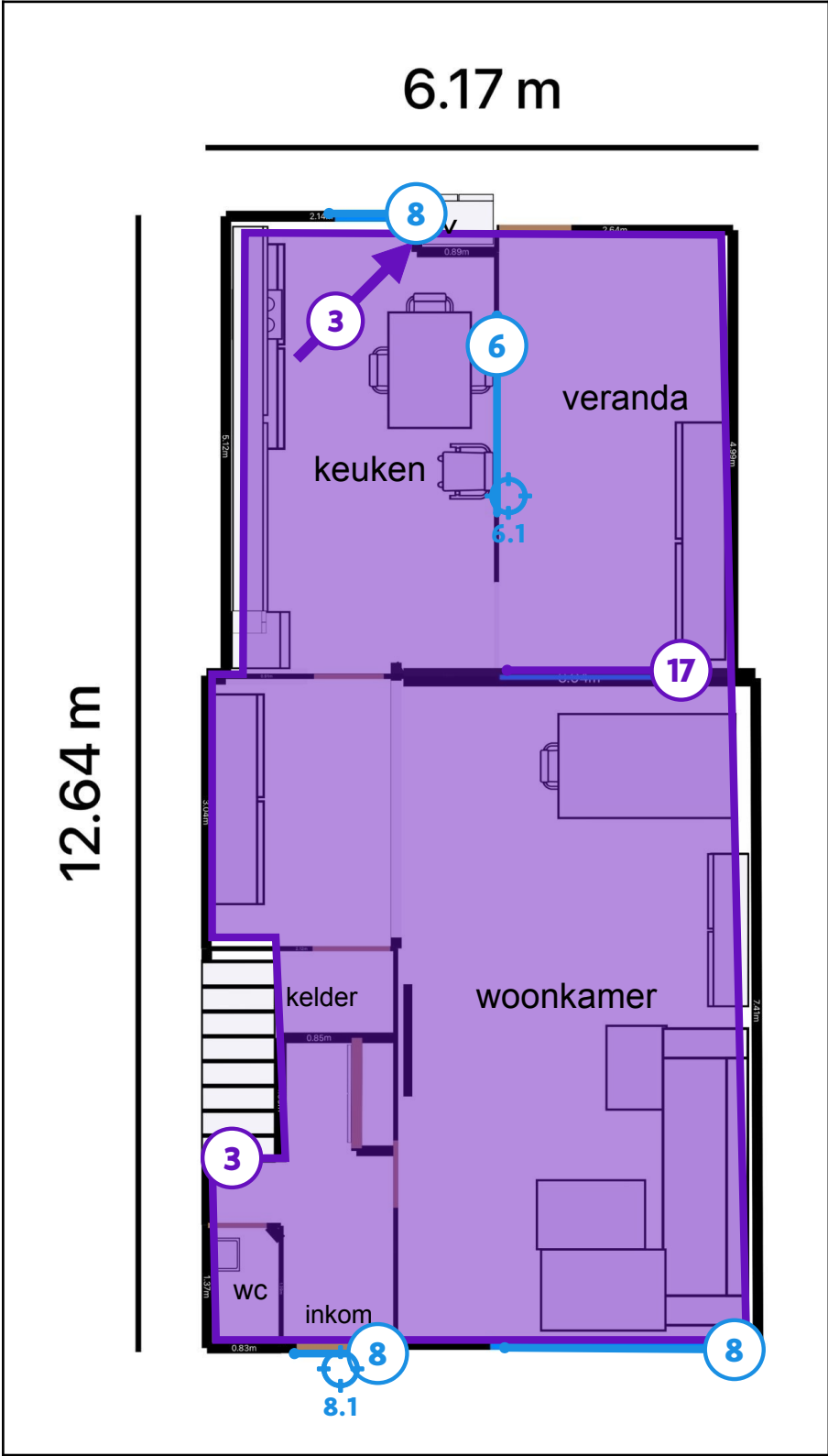
Legende van plan 1.2: Gelijkvloers
