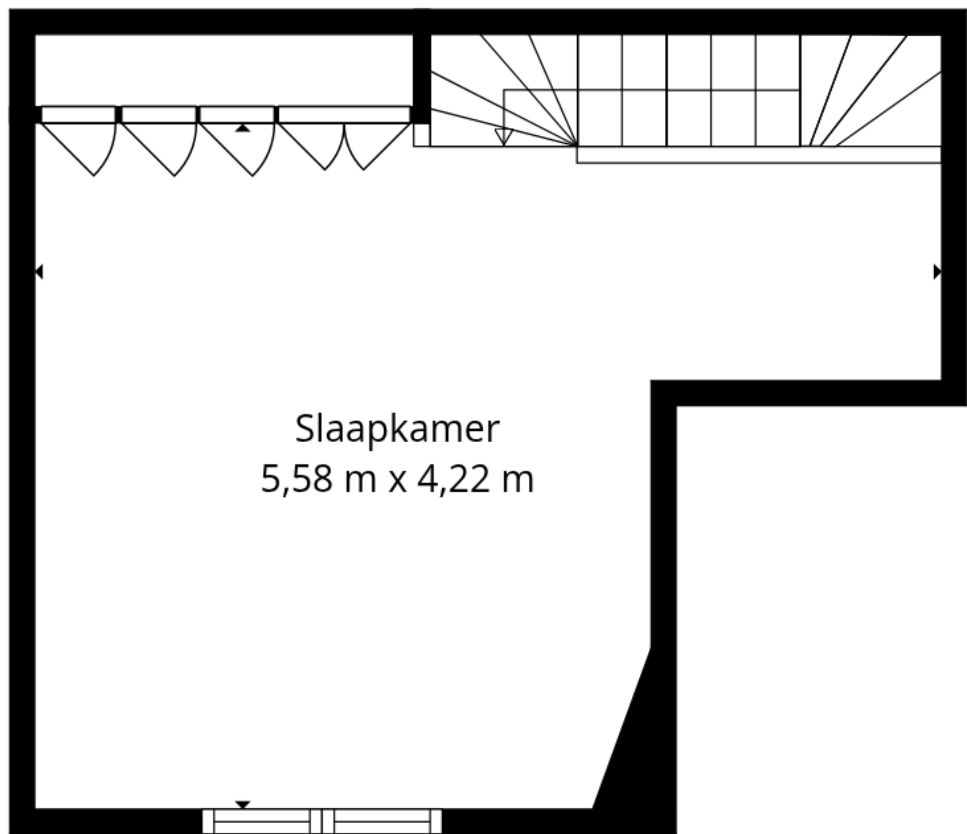
2e Verdieping
