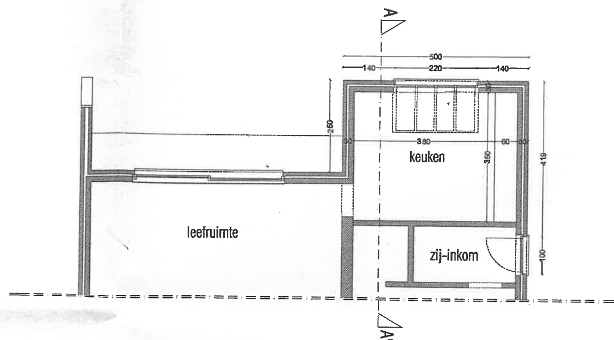
GRONDPLAN BESTAANDE TOESTAND
