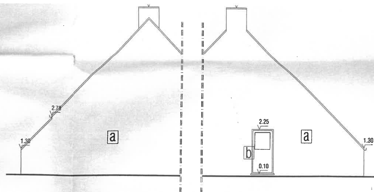
ZIJGEVEL LINKS + RECHTS BESTAANDE TOESTAND
