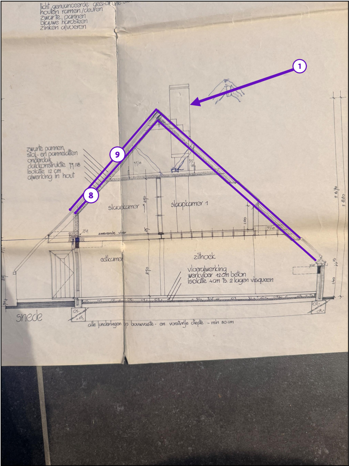
Legende van plan 1.6: Doorsnede
