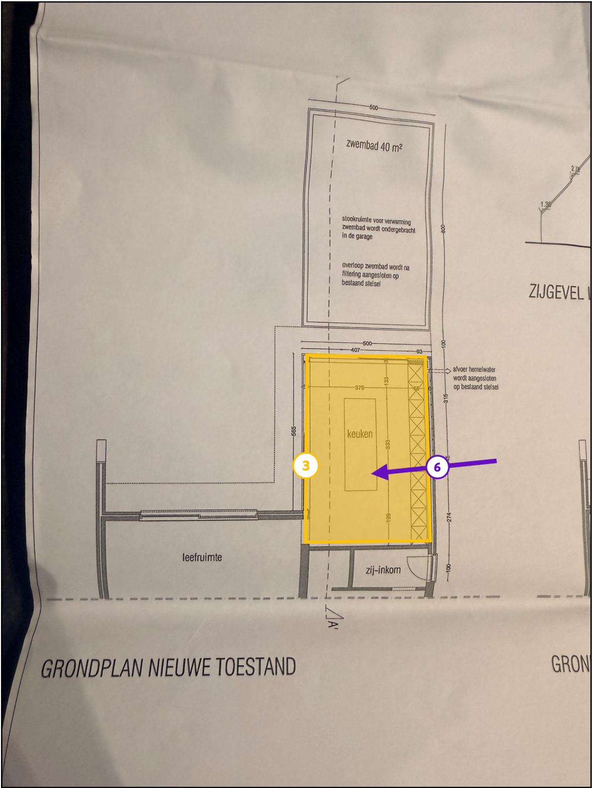
Legende van plan 1.5: Aanbouw keuken
