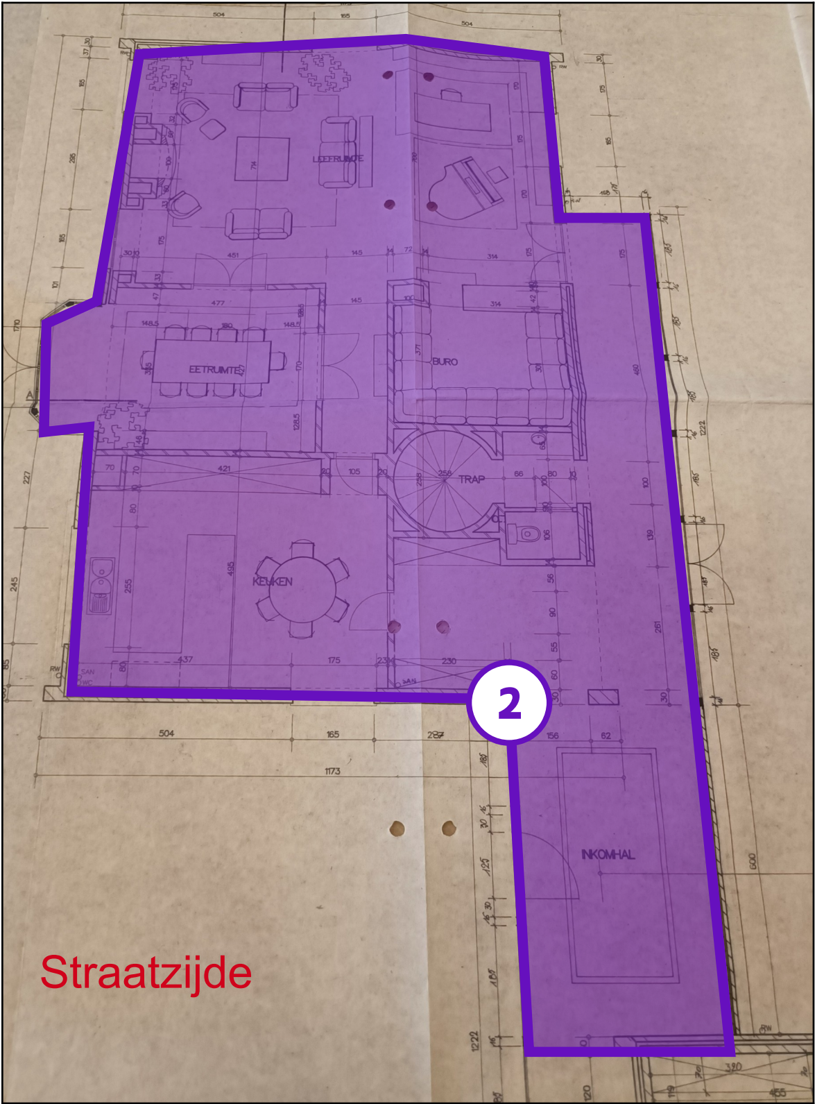
Legende van plan 1.10: Gelijkvloers vleugel zuid
